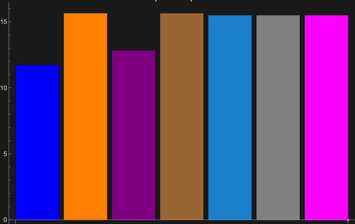
Норма L1 при t = 6
