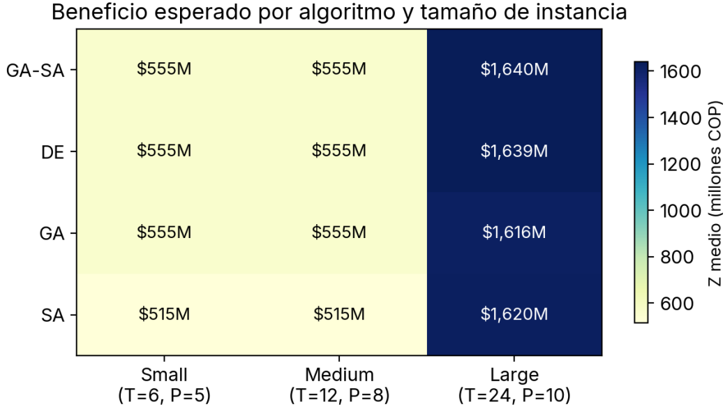
Figura 13: Beneficio esperado Z por algoritmo y tamaño de instancia. El gradiente de color permite identificar que las diferencias entre algoritmos son marginales dentro de cada tamaño, mientras que el efecto del tamaño de instancia domina la variabilidad. Las instancias Large generan beneficios del orden de 10^9 COP.
