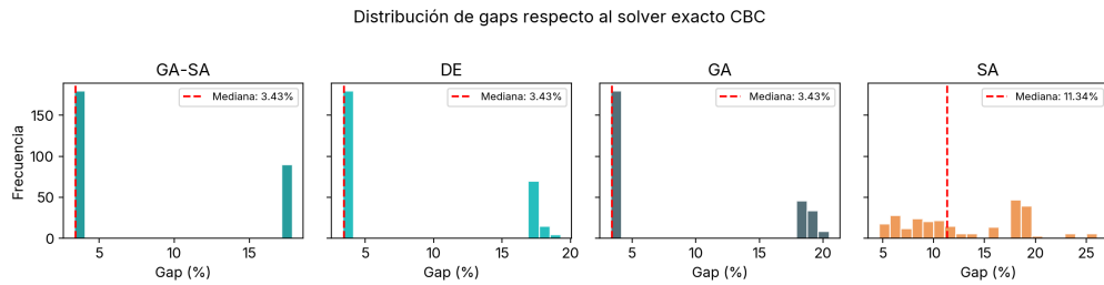
Figura 14: Distribución de gaps respecto al solver exacto CBC. GA-SA y DE concentran sus resultados en la misma zona central (mediana \approx 3.43\% y cola alta asociada a instancias Large), mientras SA exhibe mayor dispersión y peores colas de gap.
