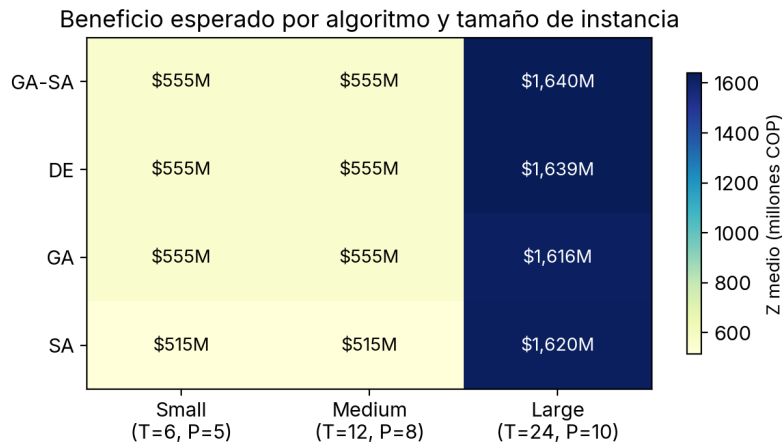
Figura 10: Heatmap de Z medio por algoritmo y tamaño de instancia
