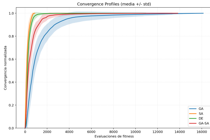
Figura 6: Convergence profiles normalizados
