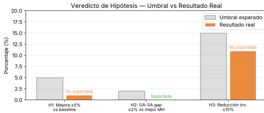
Figura 14: Veredicto de hipótesis — umbral vs resultado real
