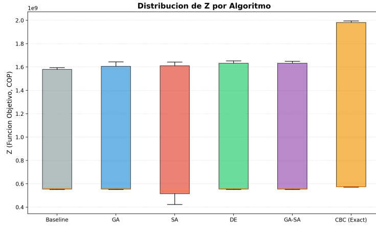
Figura 2: Boxplot de fitness por algoritmo
