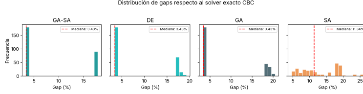
Figura 11: Distribución de gaps por algoritmo
