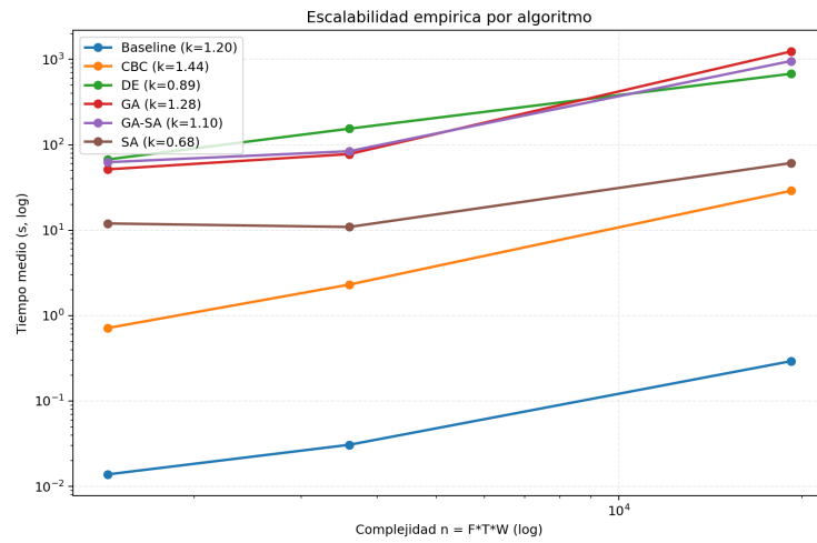
Figura 7: Escalabilidad empírica log-log
