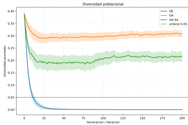
Figura 8: Diversity profiles por algoritmo
