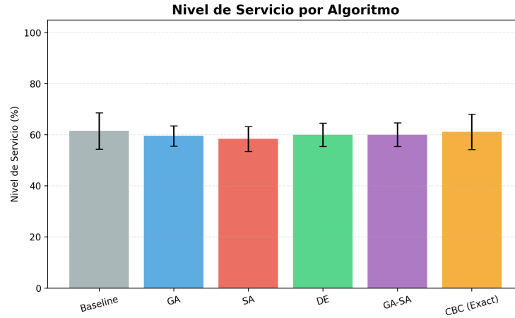
Figura 4: Nivel de servicio por algoritmo
