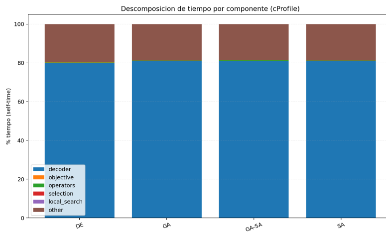
Figura 9: cProfile breakdown por componente
