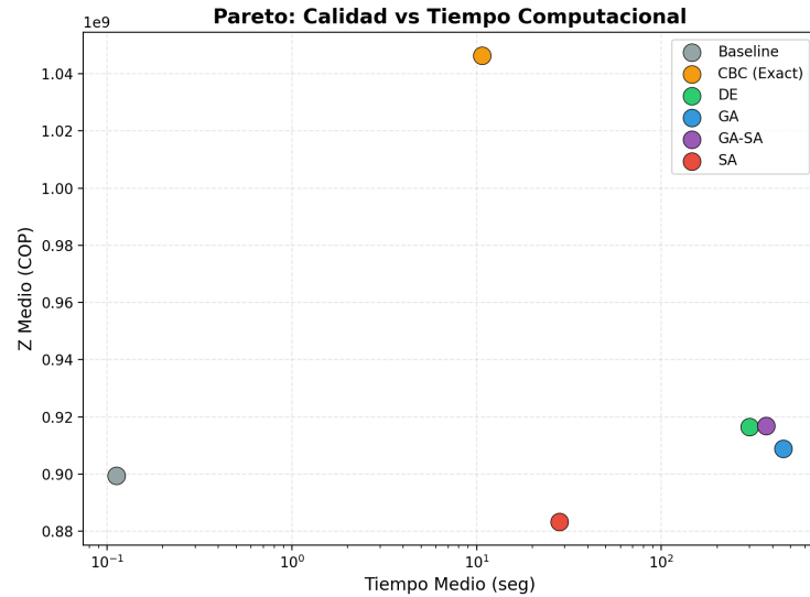
Figura 3: Pareto calidad vs tiempo
