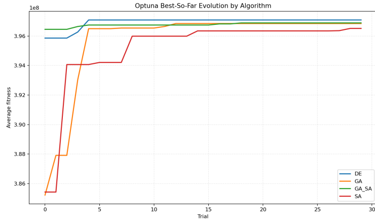
Figura 1: Evolución del score de Optuna durante calibración
