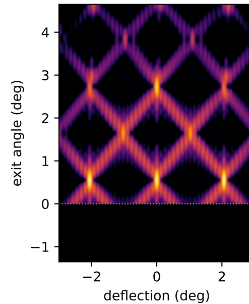
I_{00} = 0.0000
