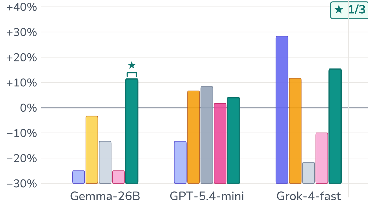
ALFWorld (OOD)
