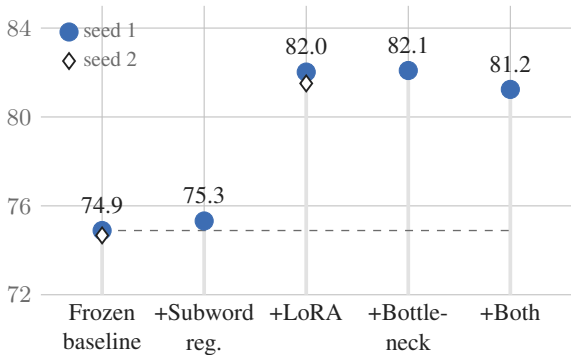
Labeled F1 (%)
