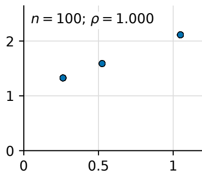
Softmax + bias
