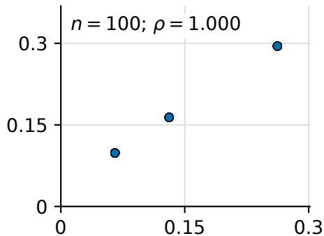
Softmax + bias
