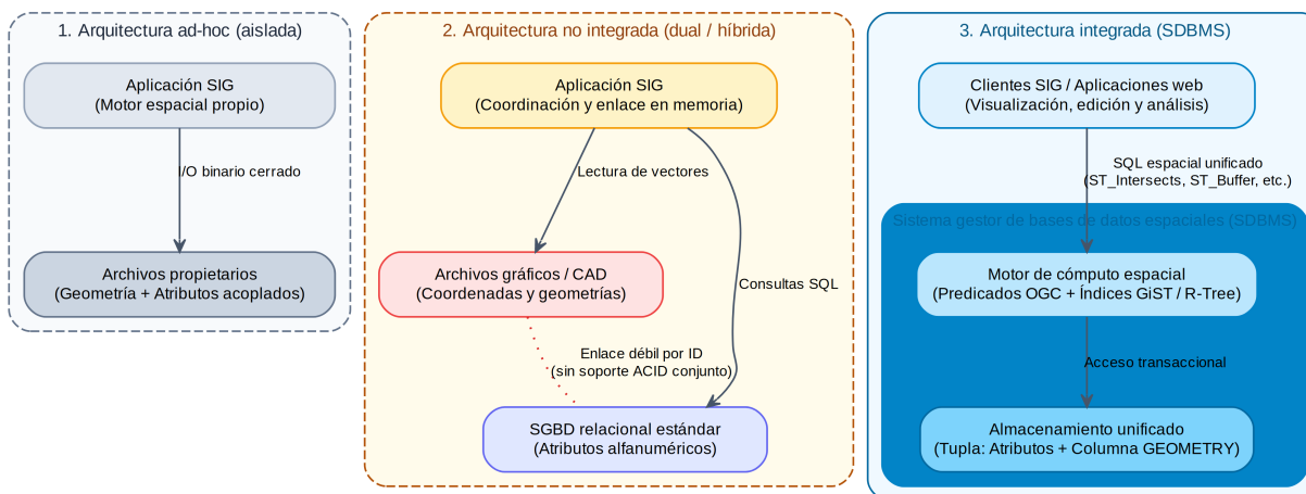
Figura 6.7: Evolución de las arquitecturas de integración entre SIG y bases de datos.
