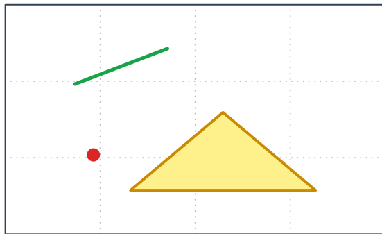
GeometryCollection (Heterogénea)
