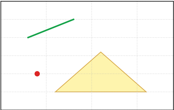
GeometryCollection (Heterogénea)
