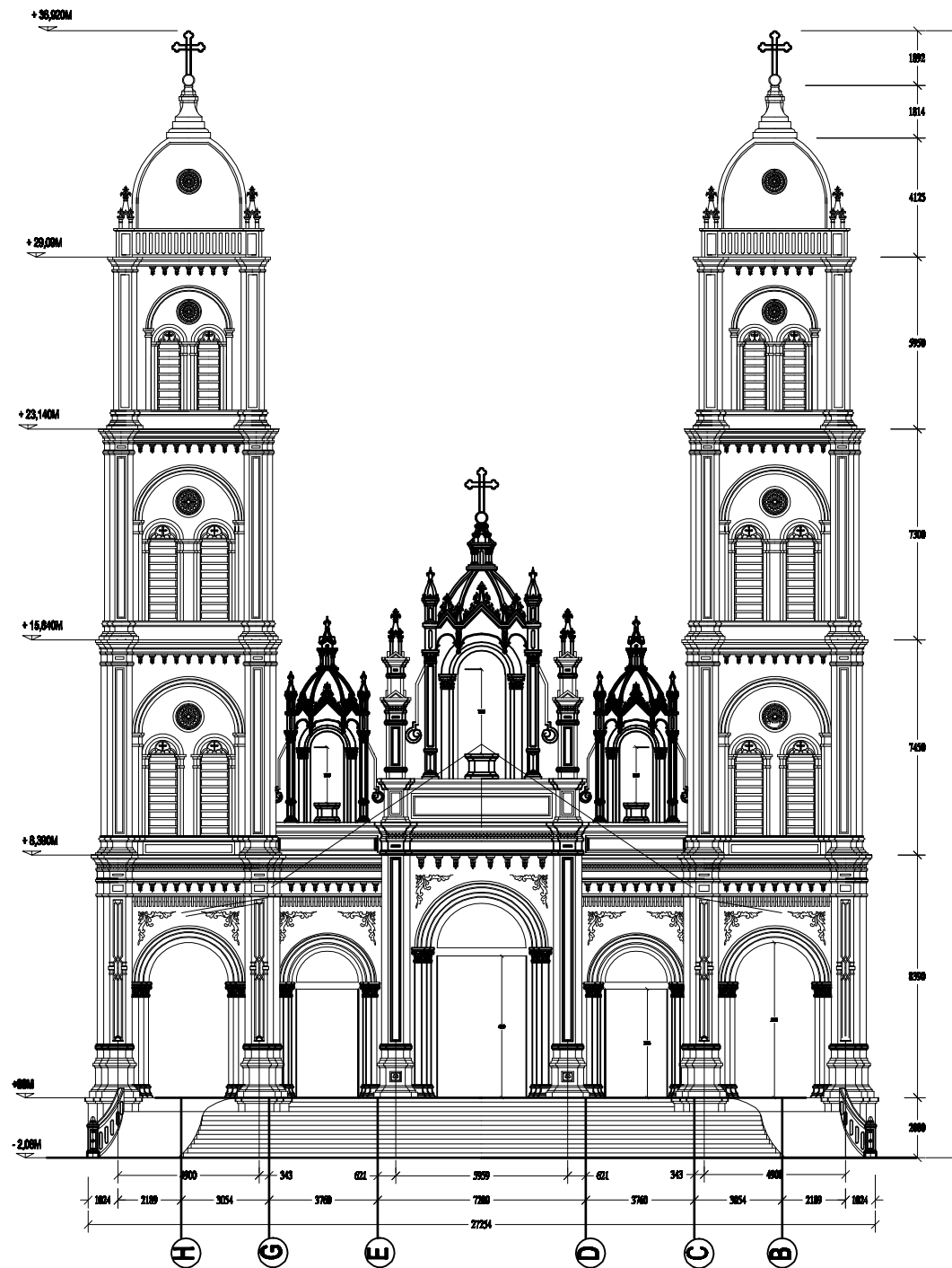
MẶT ĐỨNG CUỐI NHÀ THỜ GIÁO XỨ THẠCH BÌ
