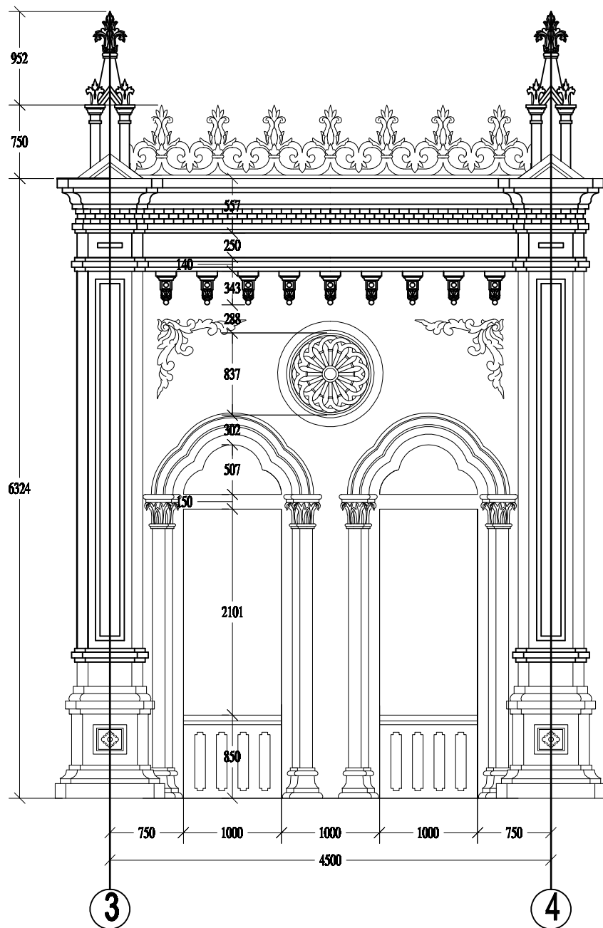
MẶT ĐỨNG TƯỜNG THÂN BÊN NGOÀI MỘT GIAN CỬA SỔ
