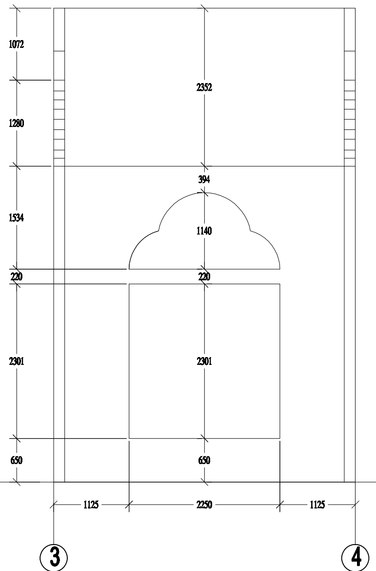
MẶT ĐỨNG TƯỜNG THÂN BÊN TRONG MỘT GIAN CỬA SỔ
