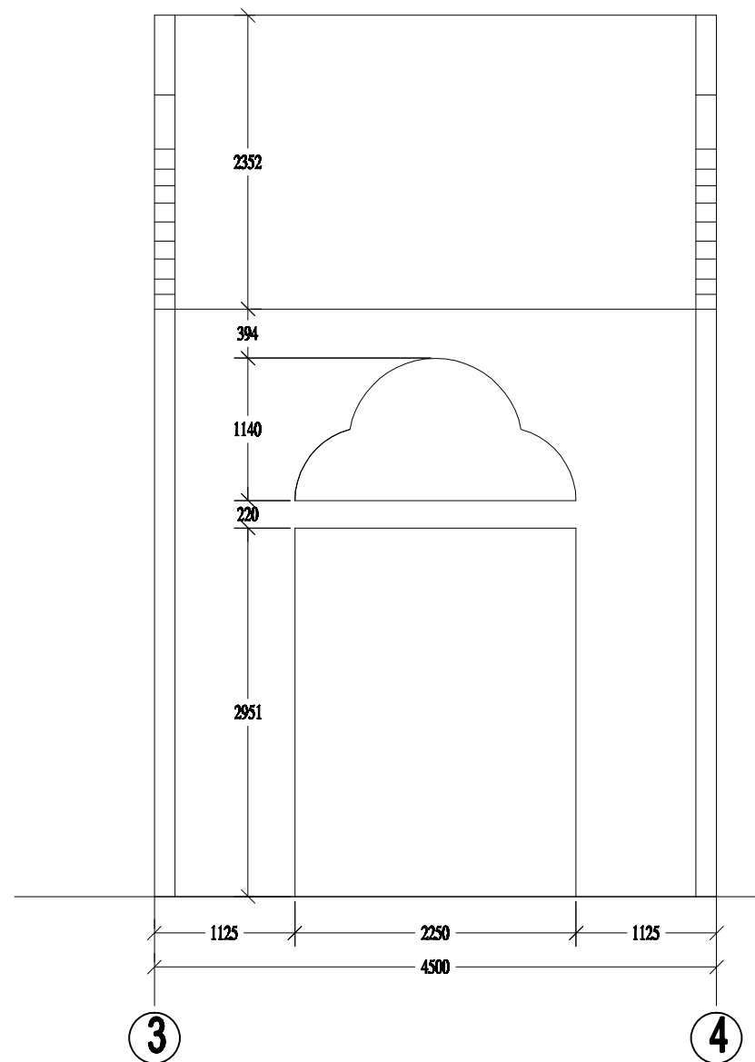
MẶT ĐỨNG TƯỜNG THÂN BÊN TRONG MỘT GIAN CỬA ĐI
