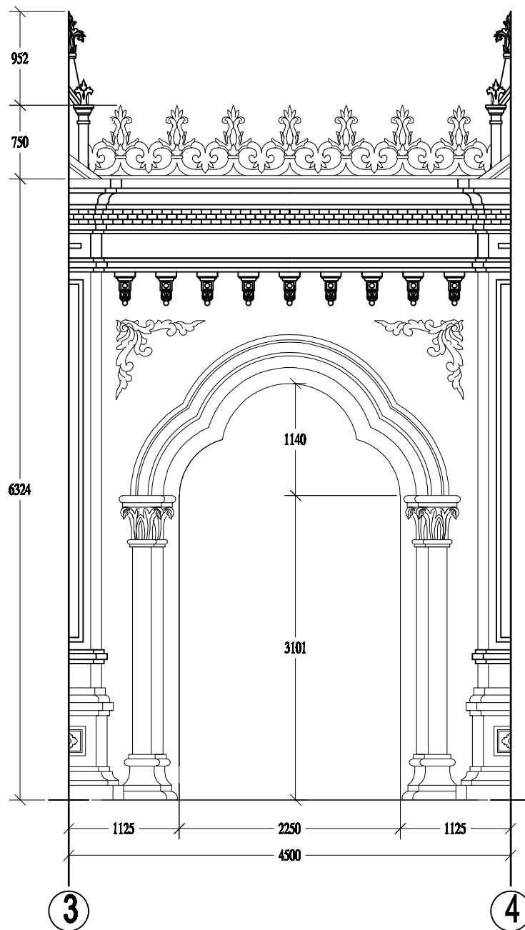
MẶT ĐỨNG TƯỜNG THÂN BÊN NGOÀI MỘT GIAN CỬA ĐI
