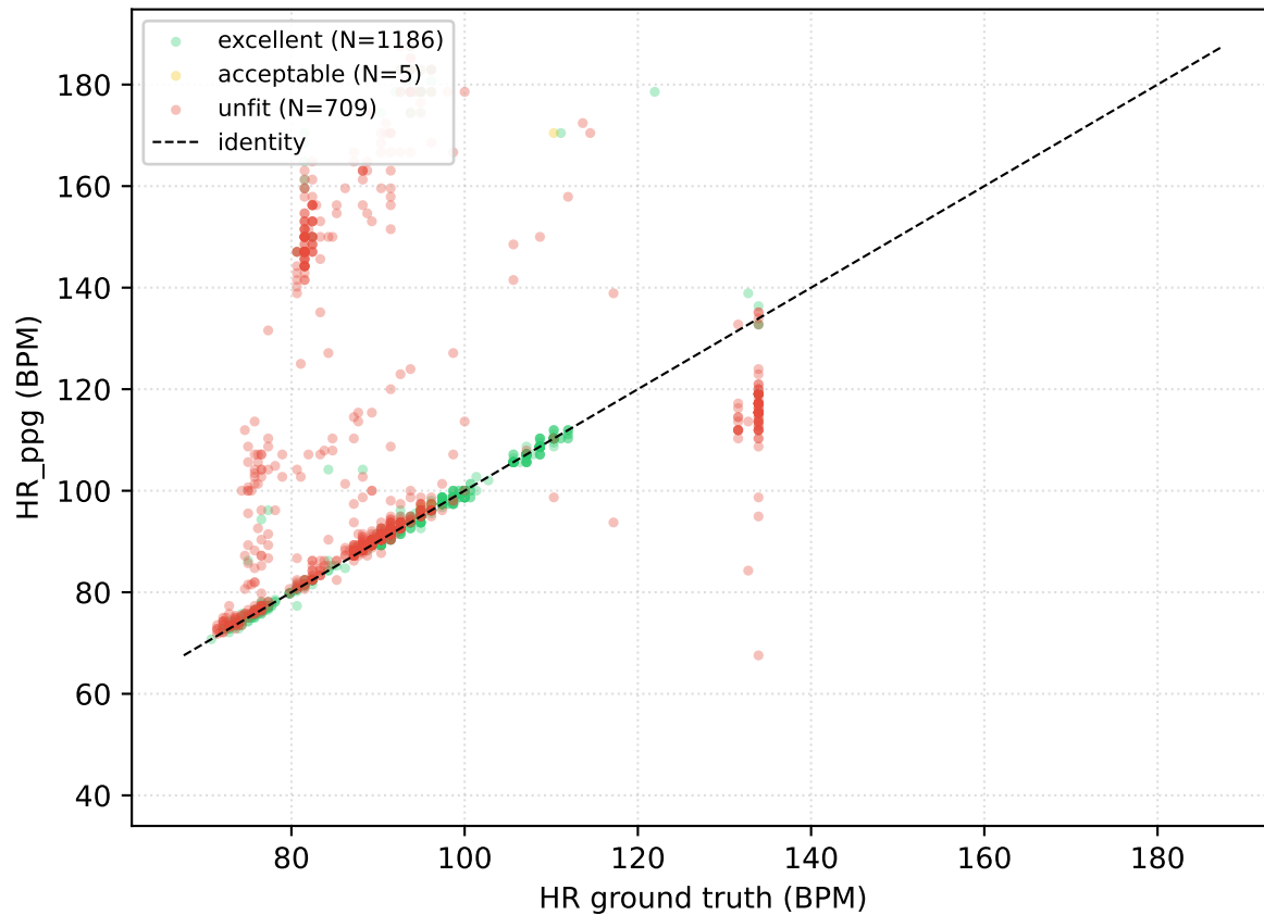
BIDMC
