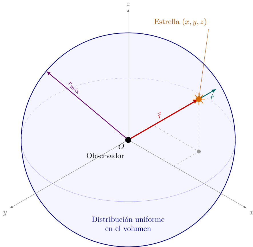
Figura 2: Geometría de la esfera y elementos vectoriales del problema. El observador está en el origen; \vec{r} localiza una estrella y R es su distancia al centro. El círculo exterior representa el contorno de la esfera de radio r_{\text{máx}} y la elipse representa su sección en el plano xy . Las líneas grises discontinuas muestran proyecciones cartesianas. La flecha \hat{r} indica la dirección radial hacia afuera y se dibuja a una escala ilustrativa.
