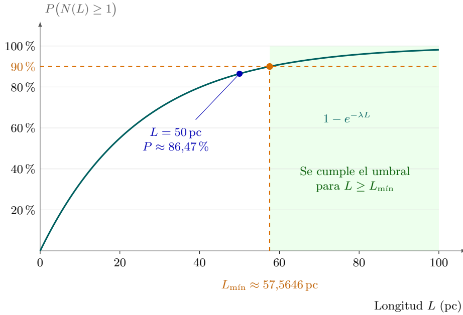
Figura 6: Probabilidad de encontrar al menos una estrella en función de la longitud observada, con \lambda = 0,04 \text{ pc}^{-1} . El cruce con el nivel del 90 % determina L_{\min} = 25 \ln 10 \text{ pc} . La zona verde señala las longitudes que satisfacen el requisito. Esta probabilidad se aproxima a 1 sin crecer linealmente, a diferencia del número esperado E[N(L)] = \lambda L .
