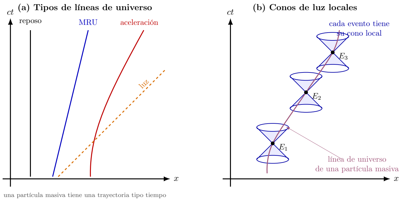
Figura 4.7: Líneas de universo y causalidad local. (a) Trayectorias de un objeto en reposo, con movimiento rectilíneo uniforme, con aceleración y de un pulso de luz. (b) Una línea de universo masiva atraviesa una sucesión de eventos, cada uno con su propio cono de luz; la trayectoria permanece siempre dentro de los conos locales.
