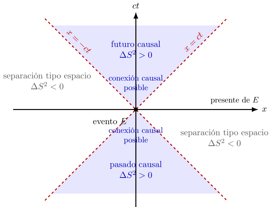
Figura 4.4: Diagrama espacio-temporal de la estructura causal respecto al evento E . Las líneas de luz x = \pm ct delimitan el cono causal: los eventos interiores tienen separación tipo tiempo y pueden estar causalmente conectados con E ; los eventos exteriores tienen separación tipo espacio y no pueden conectarse con él sin superar la rapidez de la luz.
