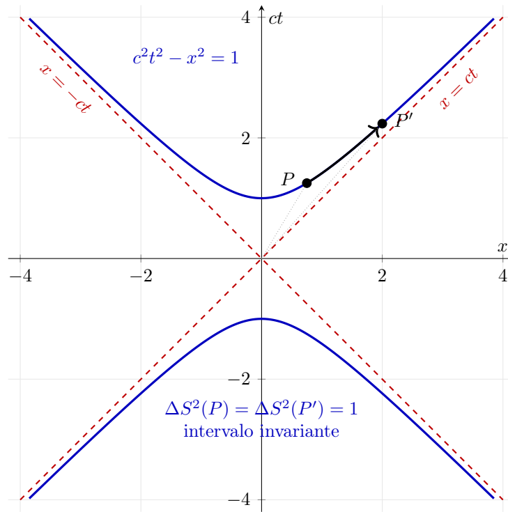
Figura 4.5: Hipérbola de intervalo espacio-temporal constante, \Delta S^2 = c^2t^2 - x^2 = 1 . Una transformación de Lorentz desplaza las coordenadas del evento de P a P' a lo largo de la misma hipérbola, sin modificar el intervalo. Las líneas de luz son sus asíntotas.
