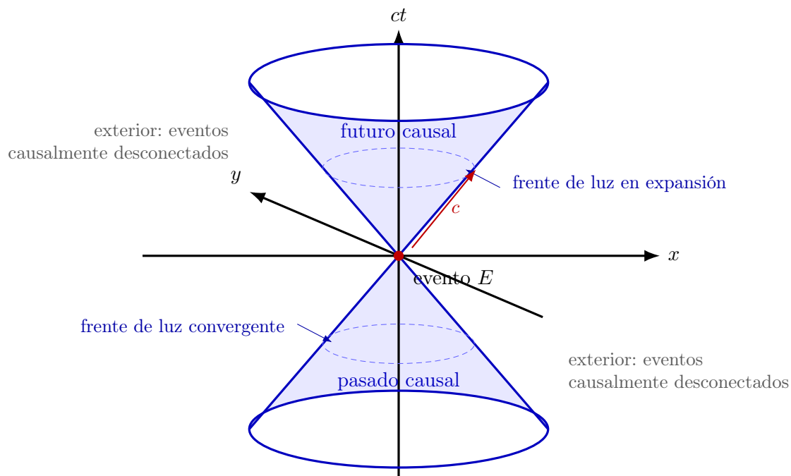
Figura 4.6: Cono de luz de un evento E considerando dos dimensiones espaciales. Cada sección horizontal representa un frente de onda circular; al apilar estos frentes en la dirección temporal se forman el cono futuro y el cono pasado. El interior contiene los eventos causalmente conectados con E , mientras que el exterior contiene separaciones tipo espacio.
