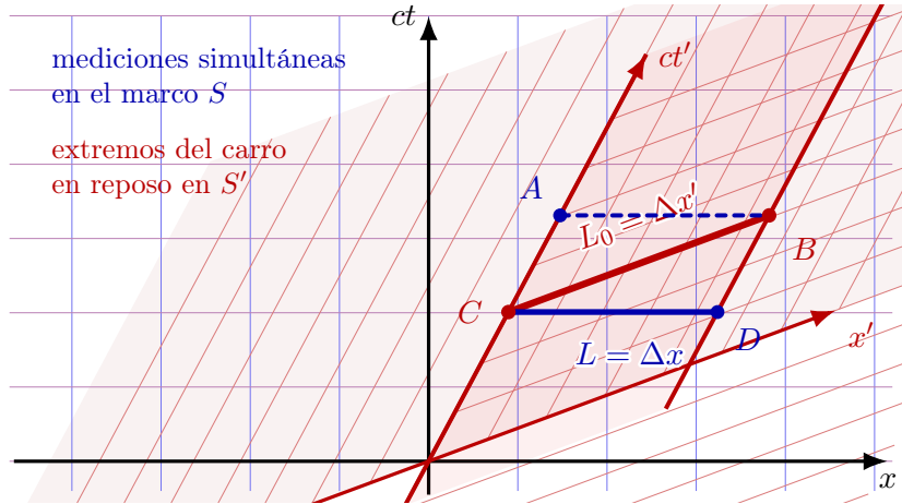
Figura 8.1: Diagrama de Minkowski para la contracción de longitudes. Los eventos C y B son simultáneos en el marco propio S' y determinan la longitud propia L_0 . En S , las mediciones simultáneas deben realizarse horizontalmente, mediante C-D o A-B , y proporcionan la longitud contraída L = L_0/\gamma .
