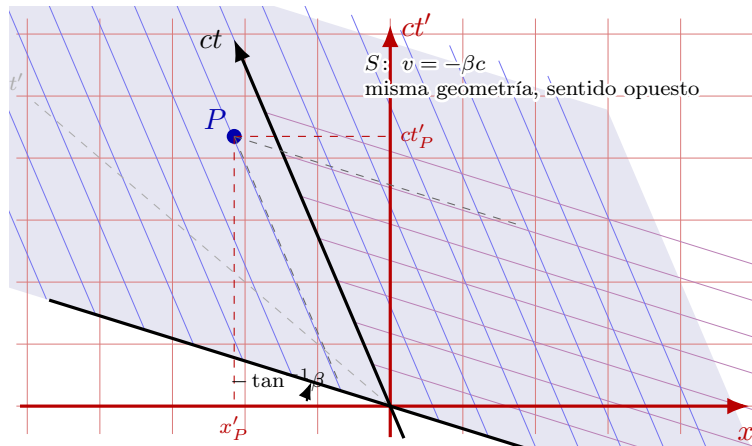
Figura 7.10: Transformación inversa tomando S' como marco base. El cambio v \rightarrow -v inclina los ejes de S en sentido opuesto, sin alterar las líneas de luz ni el evento físico representado.
