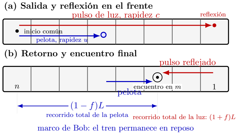
Figura 2.7: Carrera observada desde el tren. En la primera etapa, la pelota y el pulso parten del vagón n y la luz se refleja en el frente. En la segunda, el pulso regresa y encuentra a la pelota en el vagón m .
