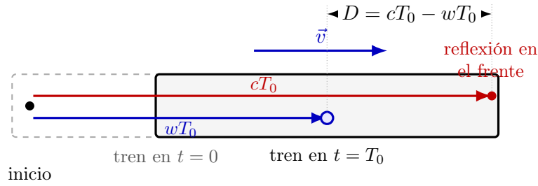
Figura 2.8: Primer intervalo visto por Alice. Desde el evento inicial hasta la reflexión, la pelota recorre wT_0 y el pulso recorre cT_0 ; la diferencia entre ambos recorridos es la separación D .
