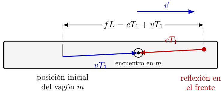
Figura 2.11: Geometría del encuentro durante T_1 . La luz recorre cT_1 hacia atrás mientras el vagón m avanza vT_1 ; ambos recorridos suman la separación inicial fL .
