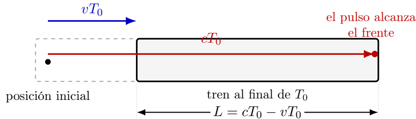
Figura 2.10: Comparación entre el desplazamiento del tren y el recorrido de la luz durante T_0 . La diferencia cT_0 - vT_0 es la longitud L del tren medida por Alice.
