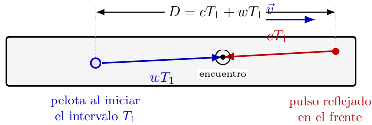
Figura 2.9: Segundo intervalo visto por Alice. Después de la reflexión, el pulso avanza hacia la izquierda y la pelota continúa hacia la derecha; la suma de ambos recorridos cubre la separación inicial D .
