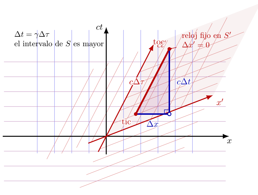
Figura 7.14: Dilatación temporal para un reloj en reposo en S' . El lado rojo inclinado une tic y toc y representa el tiempo propio \Delta\tau ; el triángulo coordenado muestra la separación espacial \Delta x y el intervalo mayor \Delta t medido desde S .
