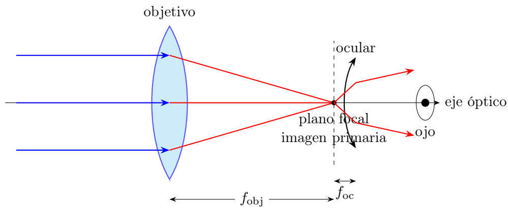
Figura 2.1: Esquema básico de un telescopio: objetivo, imagen primaria y ocular.
