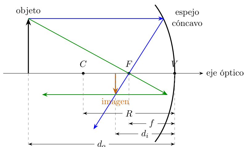
Figura 1.11: Formación de una imagen real, invertida y reducida en un espejo cóncavo.
