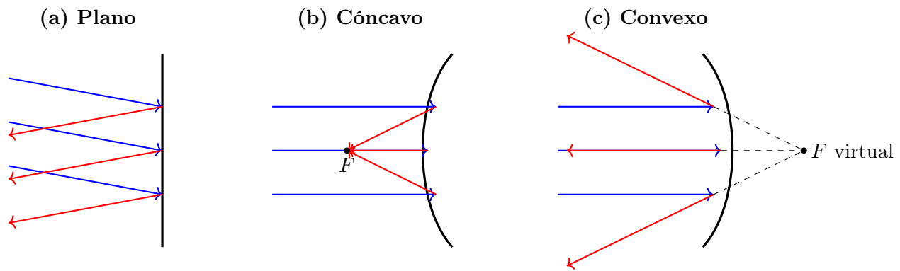
Figura 1.10: Espejo plano, cóncavo convergente y convexo divergente.
