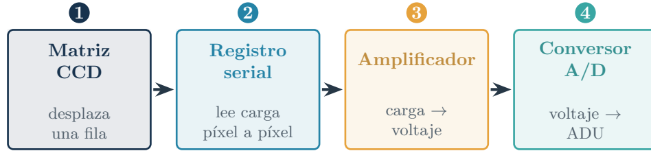
Figura 10: Cadena de lectura de un CCD, desde la matriz de carga hasta los valores digitales.
