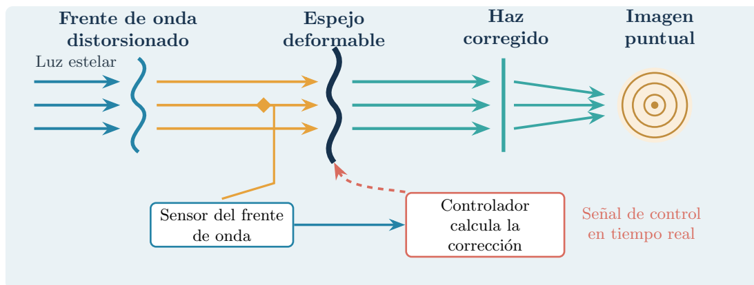
Figura 13: La óptica adaptativa mide la distorsión atmosférica y ajusta el espejo para recuperar un frente de onda regular y una imagen puntual.
