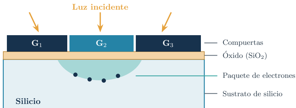
Figura 7: Corte de un píxel CCD tipo MOS: las compuertas sobre el óxido controlan el pozo donde se acumula la carga.
