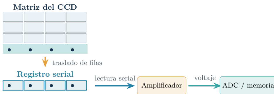
Figura 9: La carga de una fila pasa al registro serial y luego se lee píxel a píxel.
