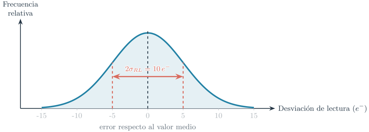
Figura 11: El ruido de lectura se manifiesta como dispersión alrededor del valor esperado.
