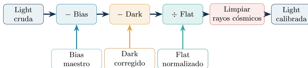
Figura 18: Secuencia de calibración: sustraer bias y dark, dividir por el flat y limpiar rayos cósmicos.
