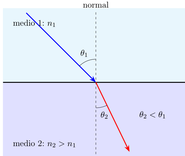
Figura 1.4: Refracción de un rayo al pasar a un medio de mayor índice.
