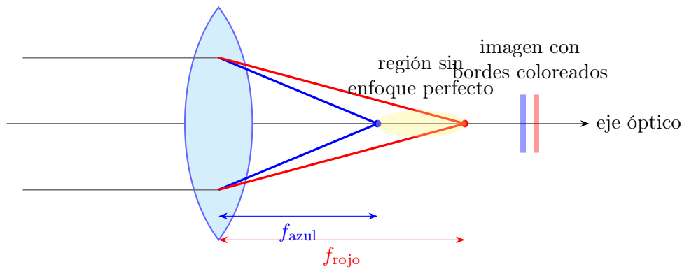
Figura 2.3: Aberración cromática longitudinal en el objetivo de un refractor.
