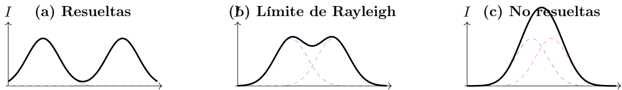
Figura 2.13: Perfiles de intensidad para dos fuentes: resueltas, en el límite de Rayleigh y no resueltas.
