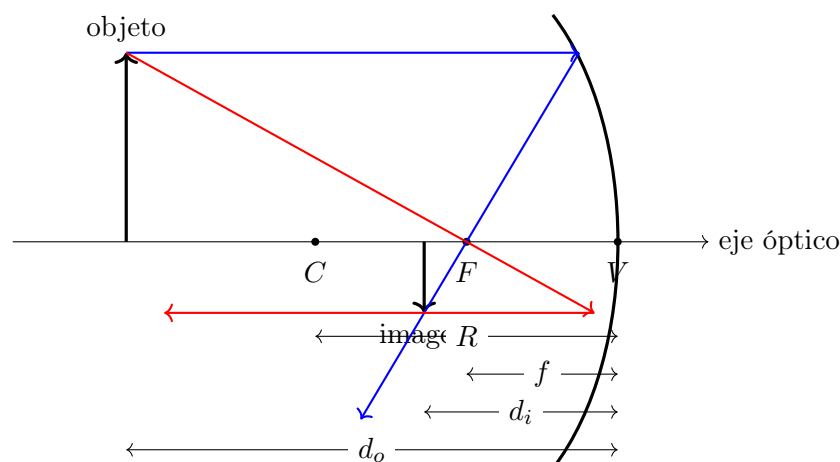
Figura 1.11: Formación de una imagen real, invertida y reducida en un espejo cóncavo.
