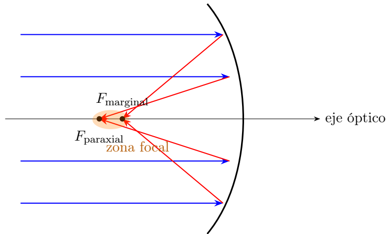
Figura 1.12: Aberración esférica: los rayos marginales y paraxiales no comparten un único foco.
