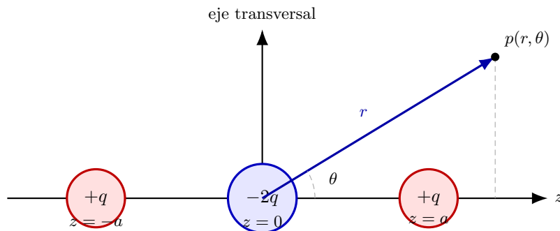
Figura 3: Geometría del cuadrupolo eléctrico lineal.
