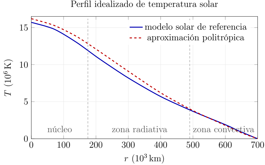
Figura 10.2: Comparación esquemática entre un perfil solar de referencia y una aproximación politrópica. El acuerdo mejora en la envoltura convectiva, donde el transporte es aproximadamente adiabático.
