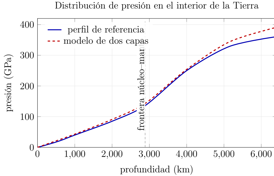
Figura 10.1: Comparación cualitativa entre un perfil terrestre de referencia y el modelo de dos capas con densidades constantes. El modelo elemental reproduce la escala de la presión central y el cambio de pendiente en la frontera núcleo-manto.
