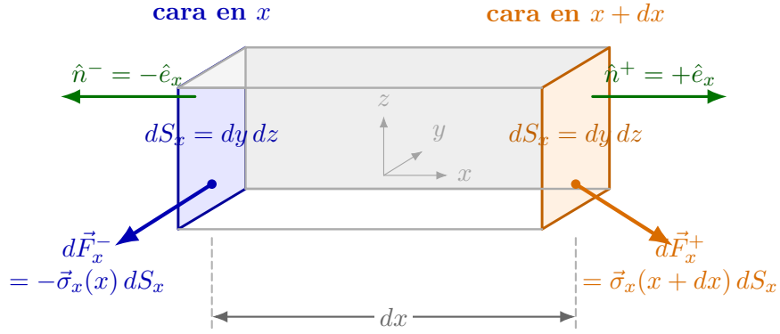
Figura 7. Fuerzas sobre las dos caras normales a x de un elemento diferencial. Las normales exteriores son opuestas: en la cara situada en x apunta -\hat{e}_x , mientras que en la cara situada en x + dx apunta +\hat{e}_x . Por ello, las fuerzas correspondientes tienen signos opuestos. Las flechas de fuerza son esquemáticas y no tienen que ser normales a las caras.
