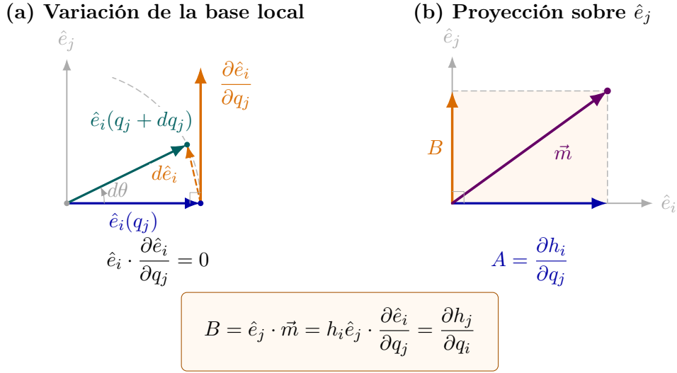
Figura 1 del Taller 6. Geometría de la proyección para i \neq j , con índices fijos. (a) Al mantener |\hat{e}_i| = 1 , su derivada es perpendicular a \hat{e}_i . La flecha discontinua representa el incremento finito; en el límite, d\hat{e}_i \simeq (\partial \hat{e}_i / \partial q_j) dq_j sigue la dirección tangente. (b) En el plano local, \vec{m} = \partial^2 \vec{r} / (\partial q_j \partial q_i) = \partial^2 \vec{r} / (\partial q_i \partial q_j) tiene componentes A y B . Al proyectar sobre \hat{e}_j , el término paralelo a \hat{e}_i desaparece y ambos desarrollos dan la misma componente B (naranja). Las variaciones y las longitudes de las flechas están exageradas; los otros argumentos de \hat{e}_i se mantienen fijos.
