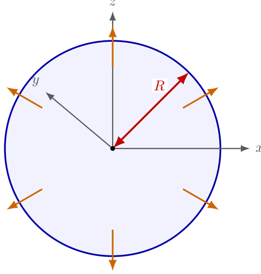
Figura 30. Corte esquemático de una esfera elástica de radio R . Las flechas indican el desplazamiento de un modo puramente radial.
