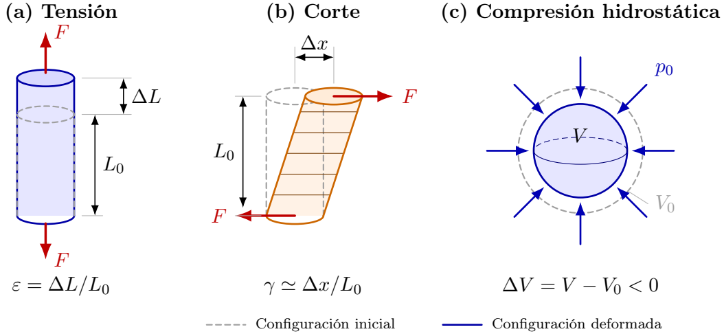
Figura 3. (a) Tensión: el cilindro se alarga en \Delta L respecto de su longitud inicial L_0 . (b) Corte: la cara superior se desplaza tangencialmente una distancia \Delta x ; para deformaciones pequeñas, \gamma \simeq \Delta x/L_0 . (c) Compresión hidrostática: la presión uniforme p_0 reduce el volumen de V_0 a V , con \Delta V = V - V_0 < 0 . Los contornos discontinuos indican la configuración inicial. Las deformaciones están exageradas para facilitar su lectura.
