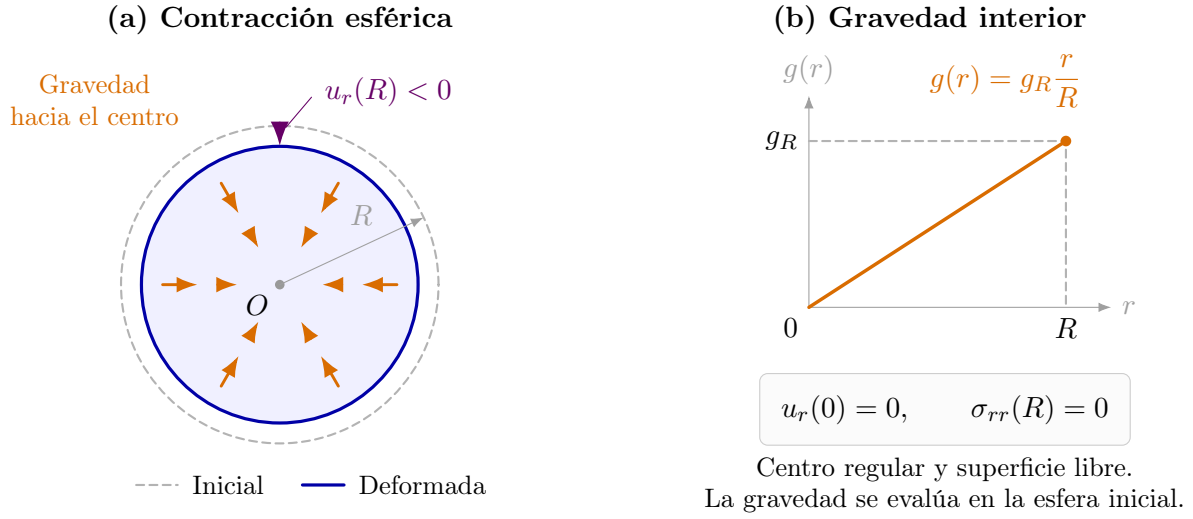
Figura 4 del Taller 7. Esfera bajo su propia gravedad. (a) Corte por el centro: las flechas gravitacionales apuntan hacia él y aumentan de magnitud con la distancia. El contorno discontinuo representa la esfera inicial y el sólido, una contracción exagerada. (b) Para densidad uniforme, la magnitud del campo gravitacional de referencia crece linealmente desde cero hasta g_R . La regularidad exige u_r(0) = 0 y la superficie libre exige \sigma_{rr}(R) = 0 .
