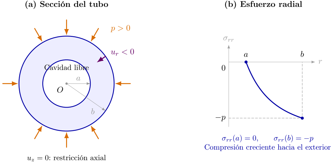
Figura 3 del Taller 7. Tubo sometido a presión externa. (a) La sección anular tiene radio interior a y exterior b ; la cavidad no está presurizada. Las flechas naranjas representan la presión exterior y la violeta indica la contracción radial. El modelo impone u_z = 0 . (b) El esfuerzo radial es nulo en la pared interior y alcanza -p en la exterior. El perfil ilustra un tubo con b/a = 2 ; la solución del texto es válida para cualquier 0 < a < b .
