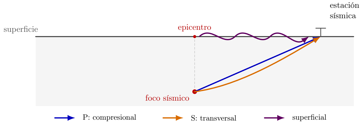
Figura 33. Esquema de las trayectorias de ondas sísmicas desde un foco hasta la superficie. Las ondas P atraviesan el interior como perturbaciones compresionales; las ondas S lo hacen como perturbaciones transversales, mientras que las ondas superficiales se propagan junto al límite del terreno.
