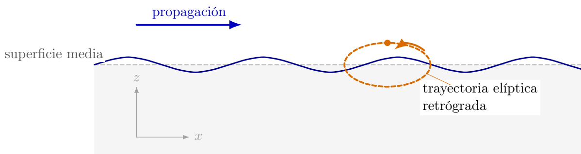
Figura 29. Esquema de una onda Rayleigh. La onda se propaga a lo largo de la superficie, mientras que una partícula superficial describe una órbita elíptica retrógrada en el plano vertical de propagación. El movimiento está ampliado.
