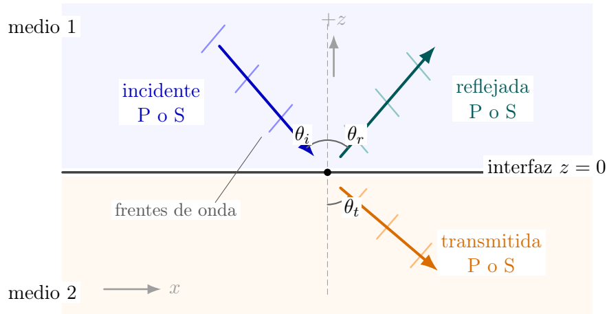
Figura 31. Reflexión y transmisión de ondas en una interfaz entre dos medios. Las flechas indican la dirección de propagación y las líneas finas, los frentes de onda; los ángulos se miden respecto de la normal. Las ondas reflejadas y transmitidas pueden ser P o S, por lo que el esquema representa una posibilidad y no todas las ramas de conversión.
