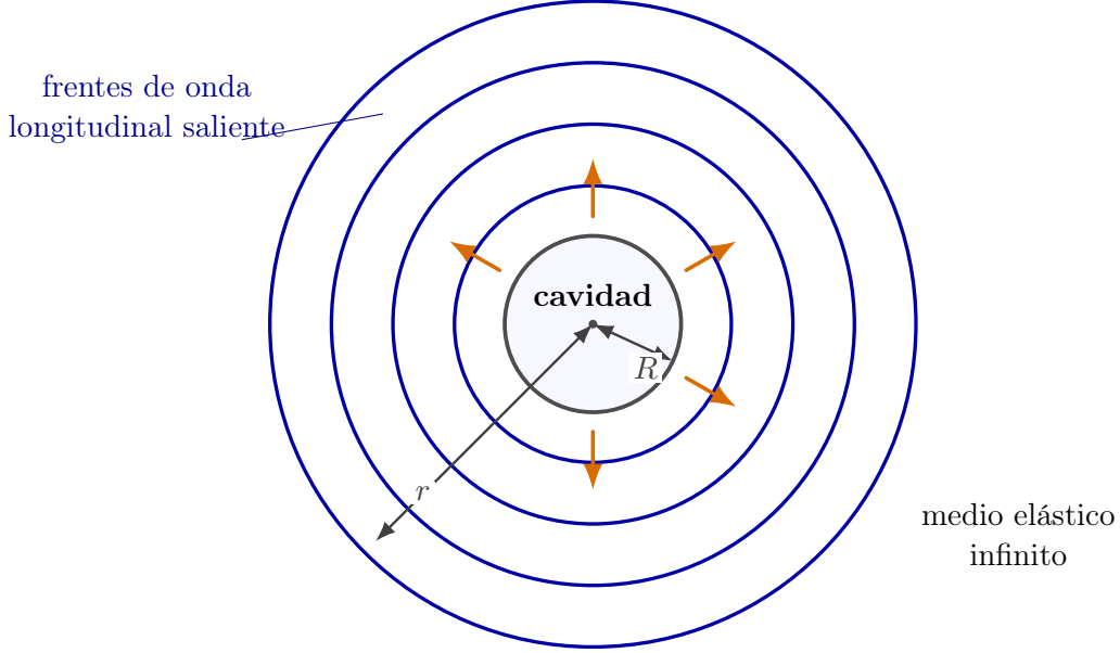
Figura 32. Corte esquemático de una cavidad esférica en un medio elástico infinito. Los círculos representan frentes de onda longitudinal que se propagan radialmente hacia el exterior; R es el radio de la cavidad y r la distancia al centro.
