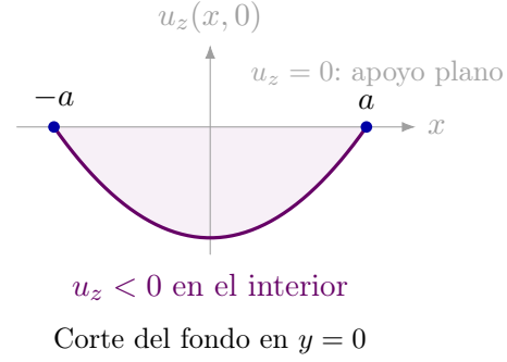
Figura 1 del Taller 7. Asentamiento sin cizalladura para \nu > 0 . (a) Corte vertical: la compresión reduce la altura y produce expansión lateral. El contorno discontinuo representa el cuerpo inicial. (b) Perfil de u_z(x, 0) en y = 0 : la referencia elegida anula el desplazamiento en x = \pm a , pero no en el interior. Por ello, el campo no satisface el apoyo sobre un fondo plano rígido. Las deformaciones y la escala vertical del perfil se exageran para facilitar su lectura.
