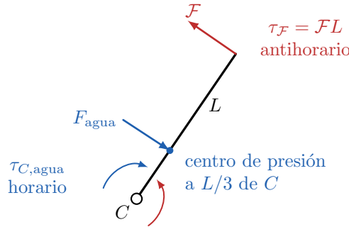
Figura 6: Diagrama de torques de la compuerta respecto a la articulación C .
