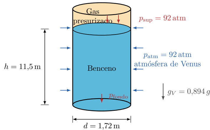
Figura 9: Tanque cilíndrico presurizado con benceno en Venus.
