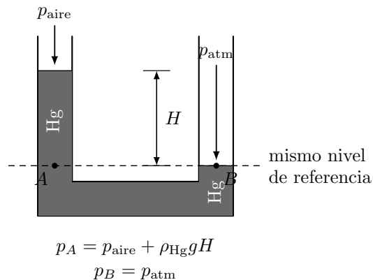
Figura 2: Balance de presión en un mismo nivel del mercurio.
