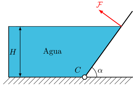
Figura 4: Geometría de la compuerta inclinada del problema 5.
