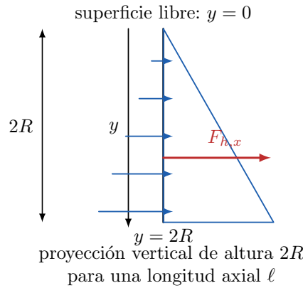
Figura 8: Proyección vertical y distribución de presión usada para calcular la fuerza horizontal.
