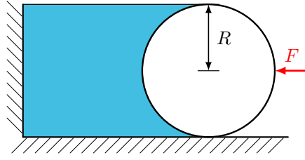
Figura 7: Cilindro sometido a la acción hidrostática del agua.
