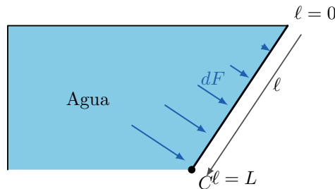
Figura 5: Distribución hidrostática sobre la compuerta, usando \ell desde la superficie libre.
