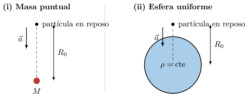
Figura 4: Comparación de la caída hacia una masa puntual y hacia una esfera uniforme.
