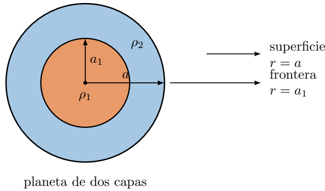
Figura 5: Modelo esférico de dos capas con densidades constantes \rho_1 y \rho_2 .
