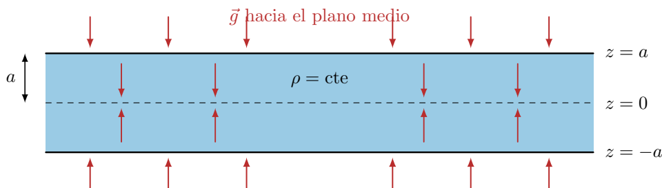
Figura 3: Placa autogravitante infinita y dirección de su campo gravitacional.
