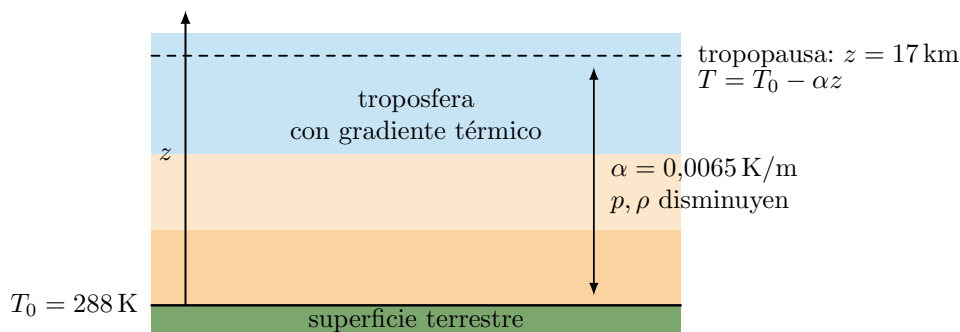
Figura 2: Modelo de atmósfera con temperatura lineal usado en el problema 3.
