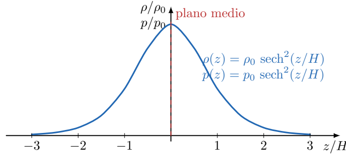
Figura 6: Perfiles normalizados de densidad y presión de la placa isotérmica.
