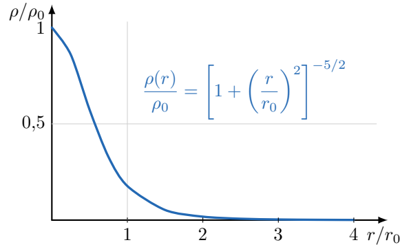
Figura 4: Distribución normalizada de densidad obtenida en la parte (a) del problema 6.
