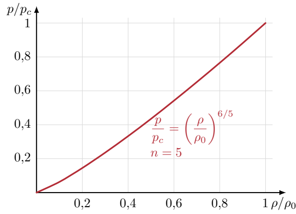
Figura 6: Relación barotrópica entre presión y densidad para la politropa de índice n = 5 .
