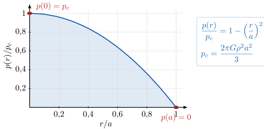
Figura 3: Perfil normalizado de presión dentro de un planeta de densidad constante.
