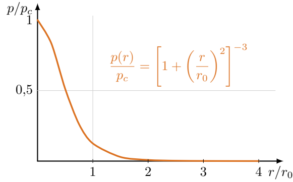
Figura 5: Perfil normalizado de presión obtenido en la parte (b) del problema 6.
