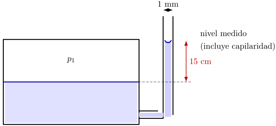
Figura 14.14: Tanque conectado a un tubo piezométrico capilar. La lectura de 15 cm combina la altura debida a la presión del tanque con la corrección capilar del tubo de 1 mm.
