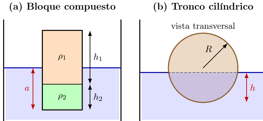
Figura 13.9: Dos configuraciones de flotación. En (a), a es la altura total sumergida del bloque compuesto. En (b), h mide la profundidad del punto más bajo del tronco respecto de la superficie del agua.
