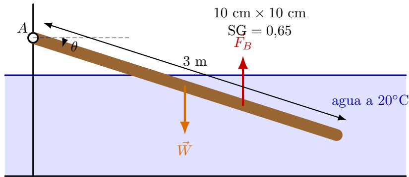
Figura 13.13: Viga uniforme articulada en A y parcialmente sumergida. El ángulo de equilibrio resulta del balance de momentos entre el peso, el empuje y la reacción de la articulación.
