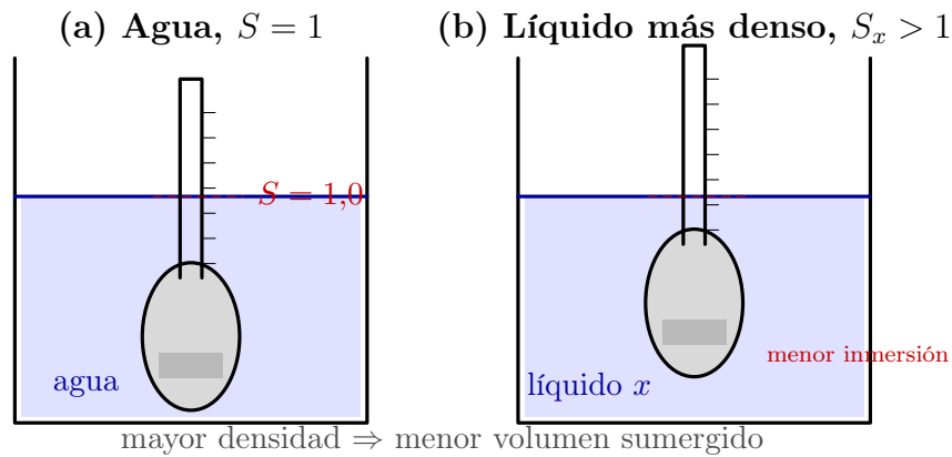
Figura 13.7: Comparación de un mismo hidrómetro en agua y en un líquido más denso. El equilibrio exige el mismo empuje en ambos casos; por ello el instrumento desplaza menos volumen y flota más alto en el líquido denso.
