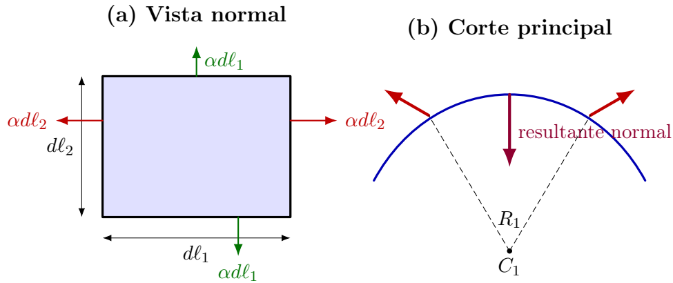
Figura 14.10: Elemento superficial alineado con las direcciones principales. Las fuerzas tangenciales en lados opuestos producen una resultante normal asociada con cada radio de curvatura.
