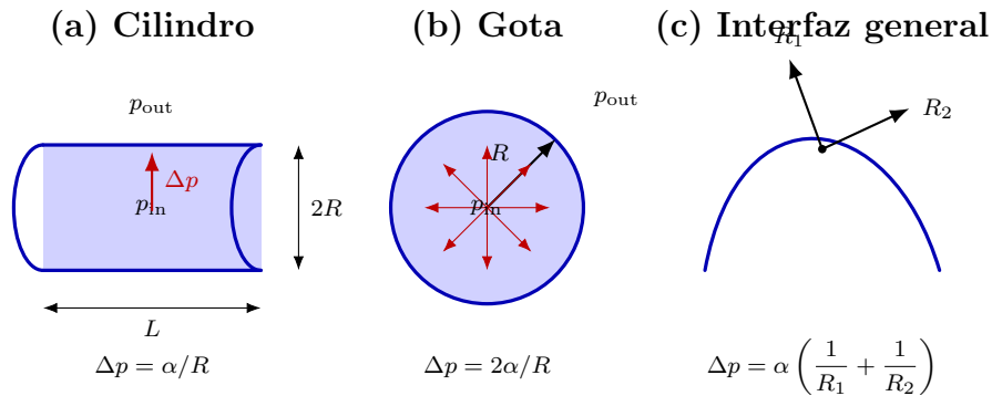
Figura 14.5: Salto de presión producido por una interfaz curva. La presión es mayor en el lado cóncavo; el valor depende de las dos curvaturas principales.
