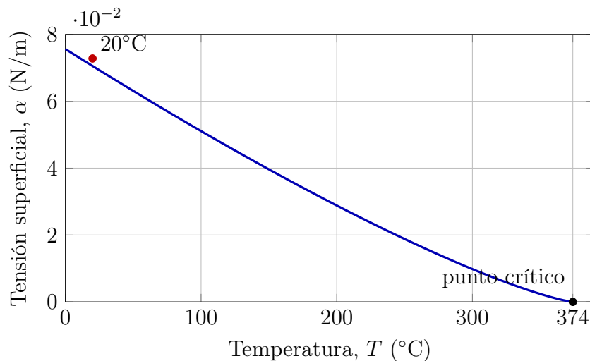
Figura 14.3: Disminución aproximada de la tensión superficial de una interfaz agua-aire limpia con la temperatura. La tensión se anula en el punto crítico.
