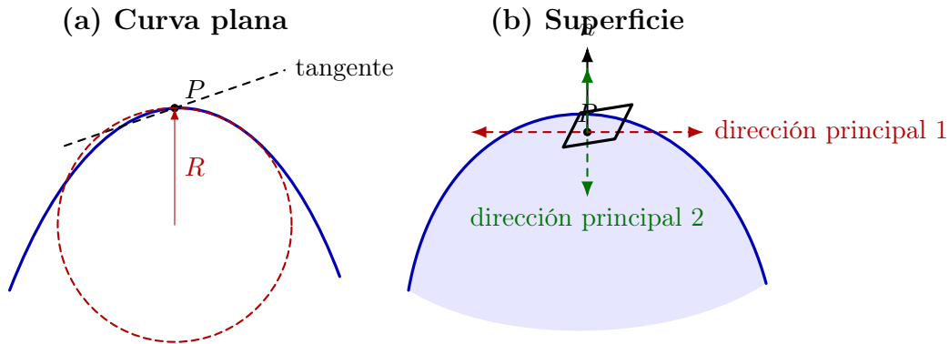
Figura 14.9: Geometría local de la curvatura. Una curva se aproxima mediante su círculo osculador; en una superficie, las curvaturas extrema y mínima definen las dos direcciones principales.
