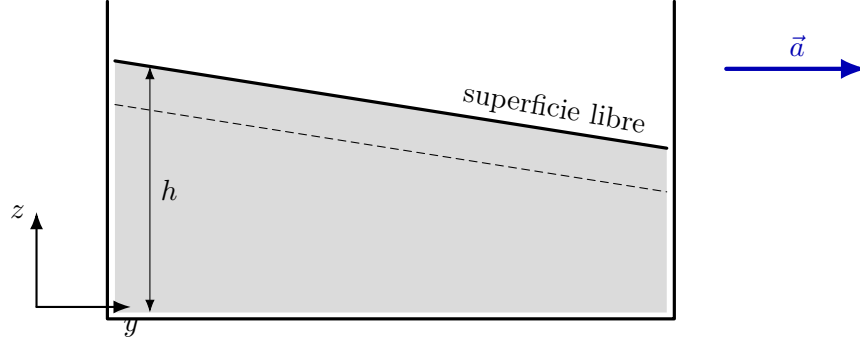
Figura 11.3: Recipiente abierto sometido a aceleración horizontal. La superficie libre es plana, asciende en el lado opuesto a \vec{a} y es perpendicular a la aceleración efectiva.
