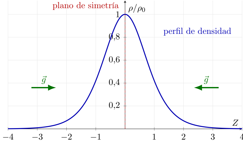
Perfil de una losa isotérmica autogravitante
