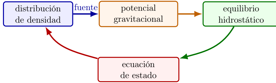
Figura 8.2: La densidad genera el potencial gravitacional mediante la ecuación de Poisson; el potencial determina el equilibrio de presión, y la ecuación de estado cierra el sistema relacionando nuevamente presión y densidad.
