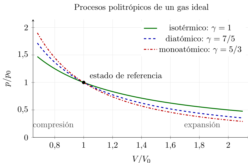
Figura 9.1: Curvas presión–volumen normalizadas para distintos índices politr3picos. Durante una compresión, la presión aumenta más rápidamente cuanto mayor es \gamma .
