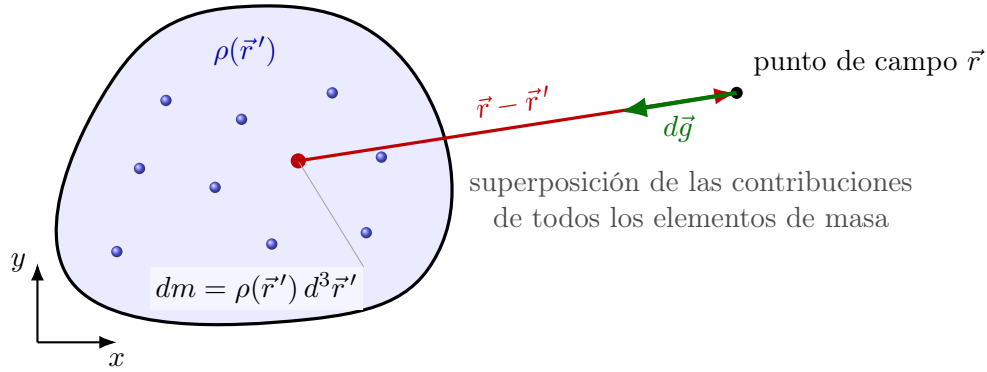
Figura 8.1: Cada elemento de masa de la distribución produce una contribución diferencial al campo gravitacional. El campo total se obtiene por superposición, integrando sobre todas las posiciones fuente \vec{r}' .
