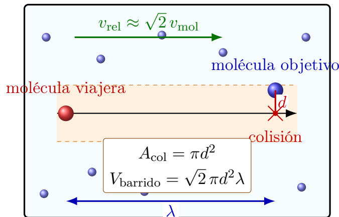
Figura 1.6: Geometría empleada para estimar el camino libre medio. Una molécula barre un cilindro efectivo de sección transversal \pi d^2 y recorre, en promedio, una distancia \lambda antes de encontrar otra molécula dentro de la región de colisión.
