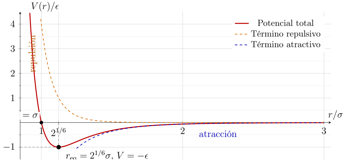
Figura 1.2: Potencial de Lennard–Jones en variables adimensionales. A distancias cortas domina el término repulsivo r^{-12} ; a distancias mayores domina el término atractivo -r^{-6} . El mínimo corresponde a la separación molecular de equilibrio.
