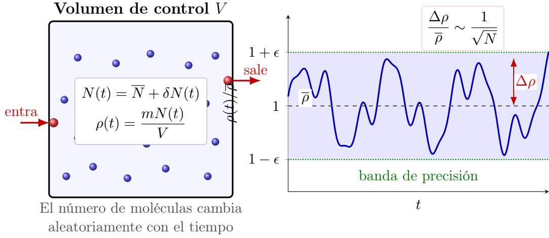
Figura 1.3: Origen estadístico de las fluctuaciones de densidad. Las moléculas entran y salen aleatoriamente de un volumen de control, haciendo que N(t) y, por tanto, \rho(t) fluctúen alrededor de sus valores medios. Al aumentar N , la amplitud relativa de las fluctuaciones decrece como N^{-1/2} .
