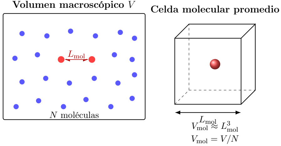
Figura 1.1: Interpretación geométrica de la longitud de separación molecular. Cada molécula se asocia con una celda de volumen promedio V/N ; al idealizarla como un cubo, su lado corresponde a L_{\text{mol}} .
