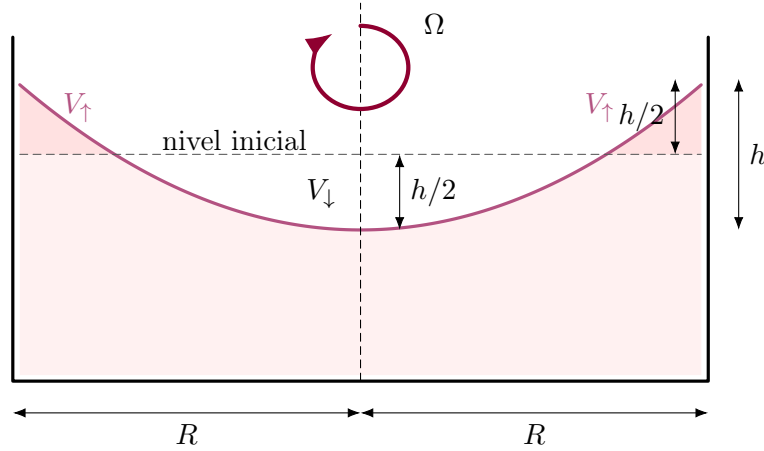
Figura 11.10: Conservación del volumen en un cilindro que rota alrededor de su eje. El volumen que desciende en la zona central es igual al volumen que asciende junto a las paredes; por ello el centro baja h/2 y los bordes suben h/2 respecto del nivel inicial.
