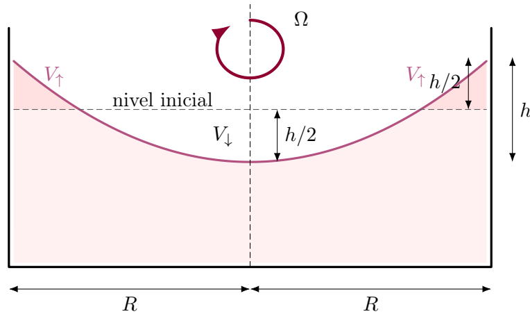
Figura 11.8: Conservación del volumen en un cilindro que rota alrededor de su eje. El volumen que desciende en la zona central es igual al volumen que asciende junto a las paredes; por ello el centro baja h/2 y los bordes suben h/2 respecto del nivel inicial.
