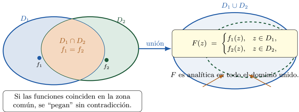
Figura 11: Visualización de la continuación analítica: dos definiciones locales f_1 y f_2 que coinciden en la intersección D_1 \cap D_2 se combinan en una única función analítica F sobre D_1 \cup D_2 .
