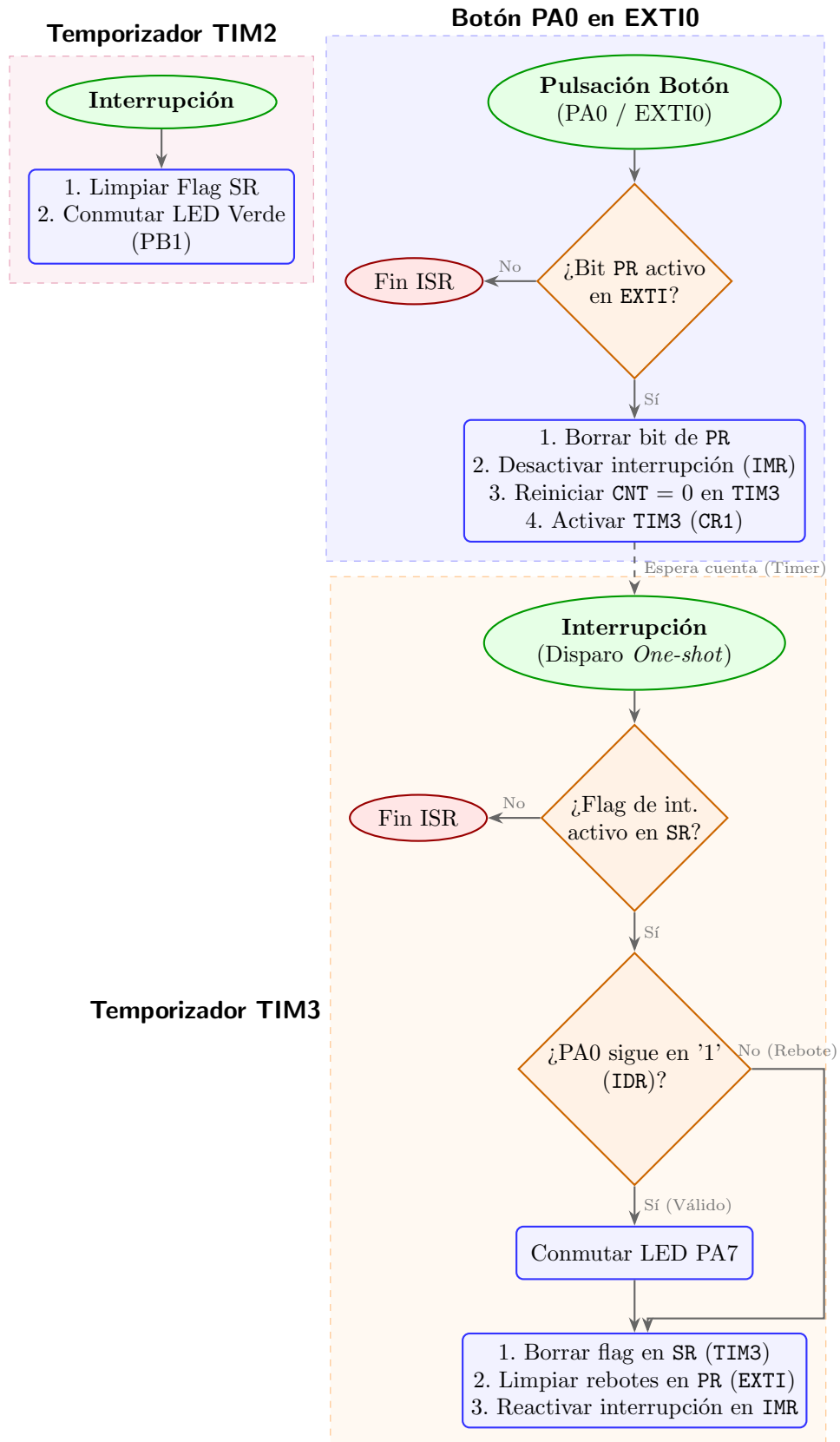
Figura 2: Diagrama de flujo funcional de las interrupciones.
