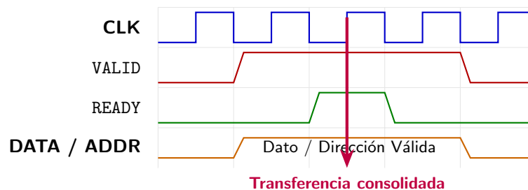
Figura 5: Sincronización por handshake en un canal AXI. La transferencia se realiza únicamente cuando VALID y READY coinciden en nivel alto durante el flanco del reloj.
