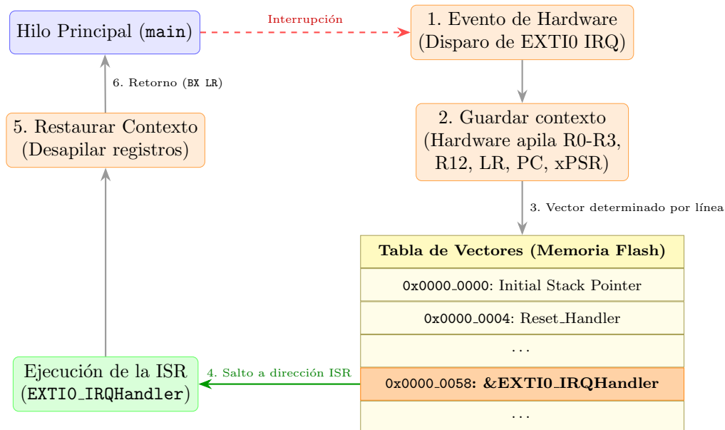
Figura 2: Mecanismo de atención a interrupciones y lectura de puntero en la Tabla de Vectores.
