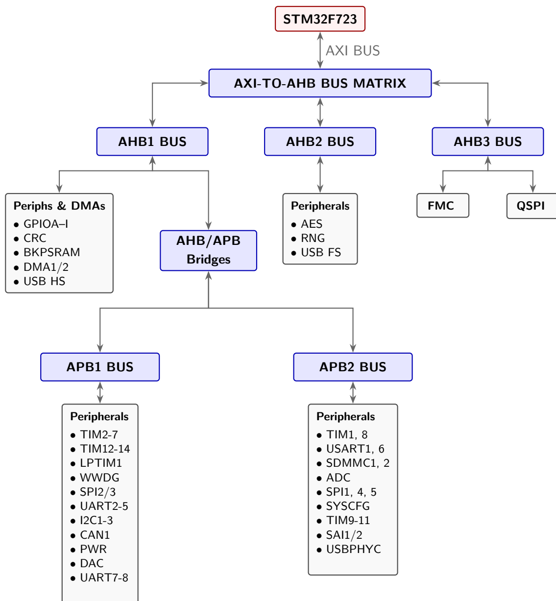
Figura 4: Interconexión del procesador y dispositivos
