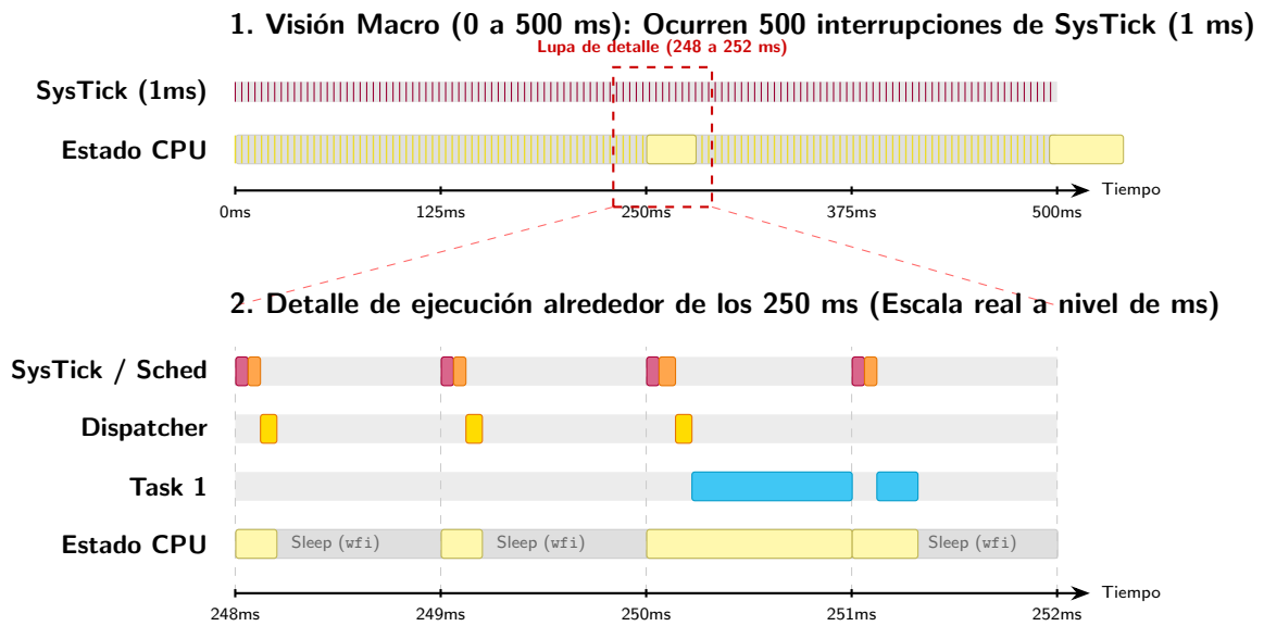
Figura 35: Detalle de ejecución de los diferentes elementos de nuestro planificador, con una tarea que tarda más de un slot
