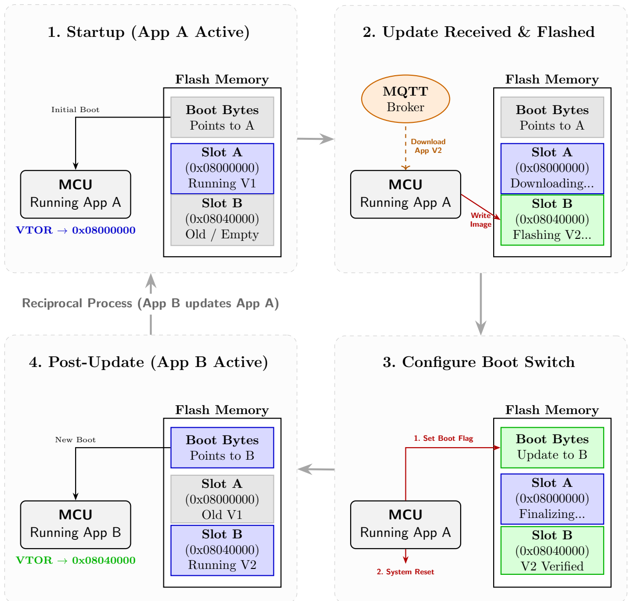
Figura 48: Diagrama de actualización A/B
