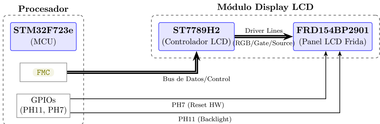
Figura 26: Diagrama de conexiones entre la MCU STM32F723, el controlador ST7789H2 y el panel LCD.
