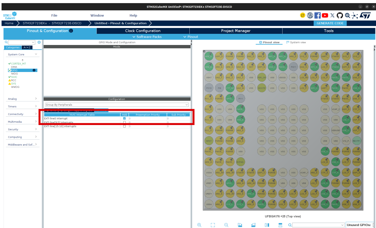
Figura 46: Activación de interrupciones para el pin de GPIO A0
