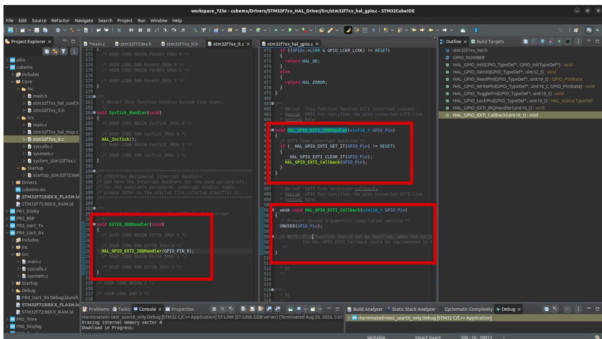
Figura 68: Estructura de las interrupciones, se ofrece mediante un callback al usuario
