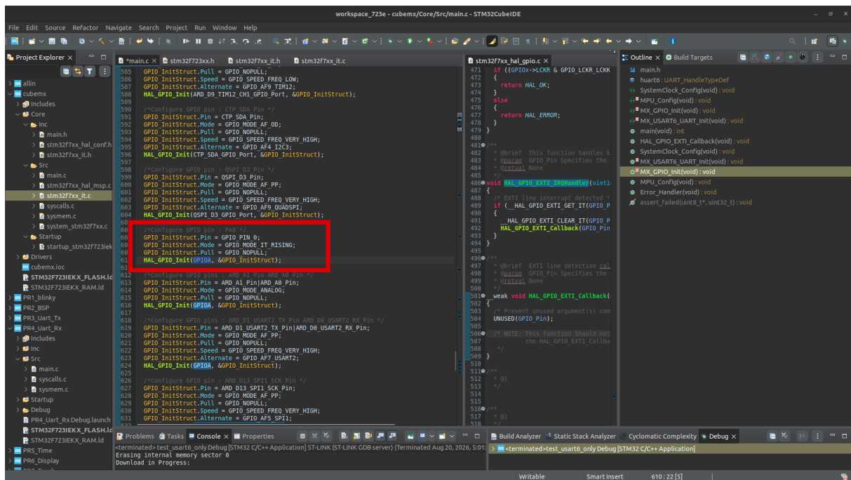
Figura 65: Configuración automática del pin para el Botón
