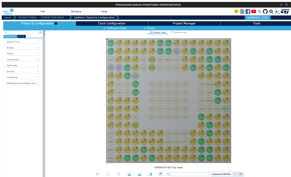
Figura 52: Disposición inicial del procesador en cubemx. Se observan todos los pines y sus funciones
