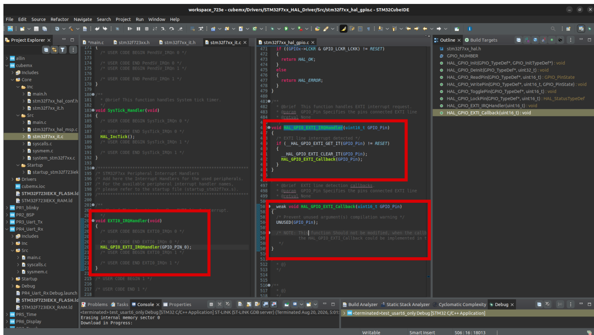
Figura 65: Estructura de las interrupciones, se ofrece mediante un callback al usuario
