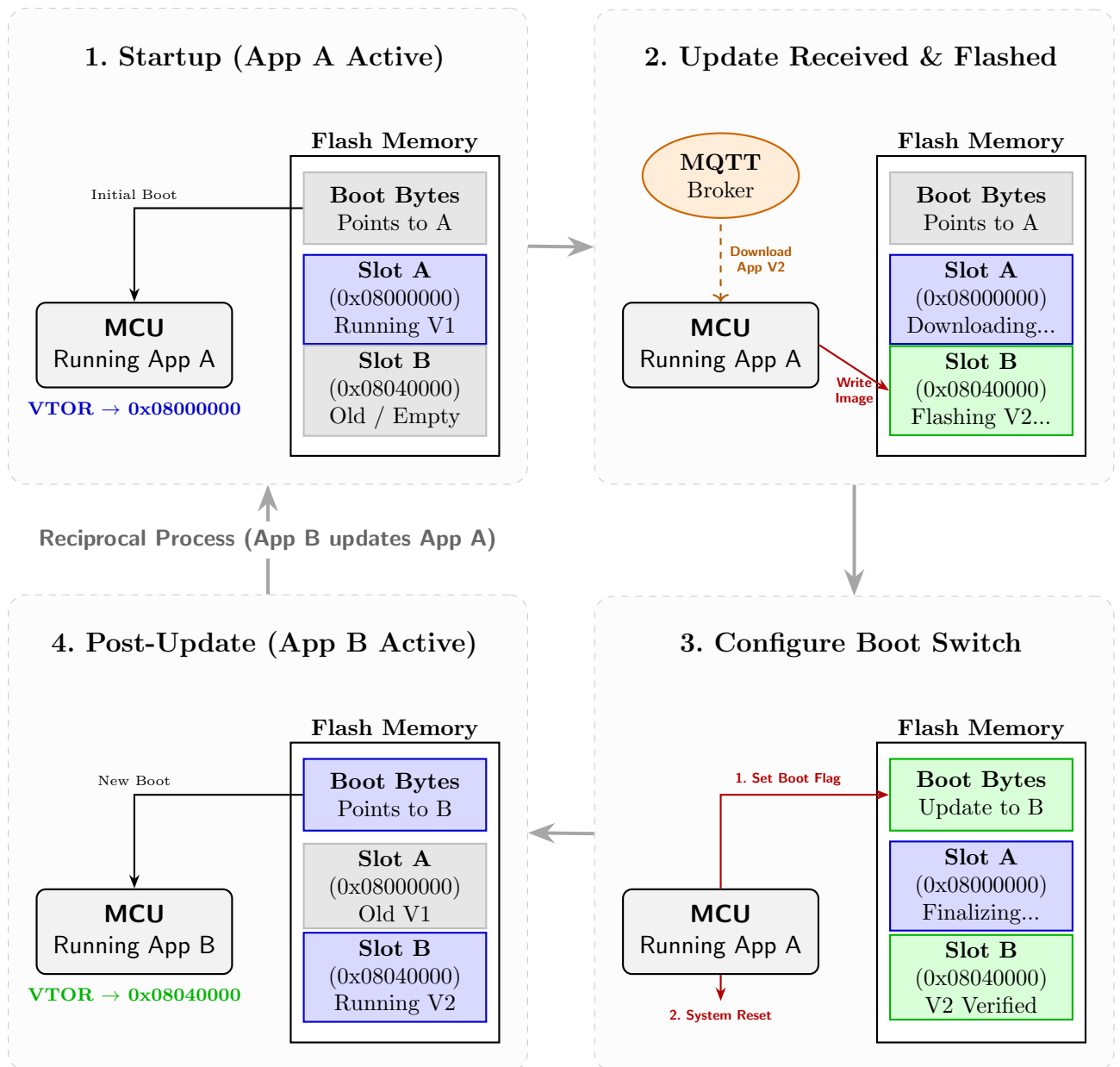
Figura 41: Diagrama de actualización A/B
