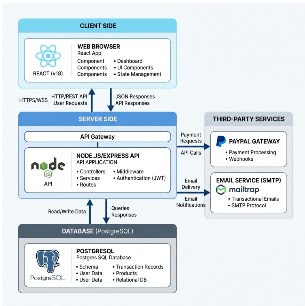
Hình ảnh 3.1: Kiến trúc tổng quan hệ thống
