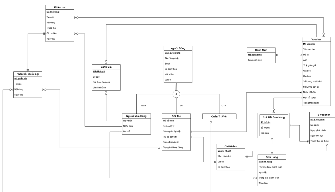
Hình ảnh 5.1: ERD hệ thống voucher
