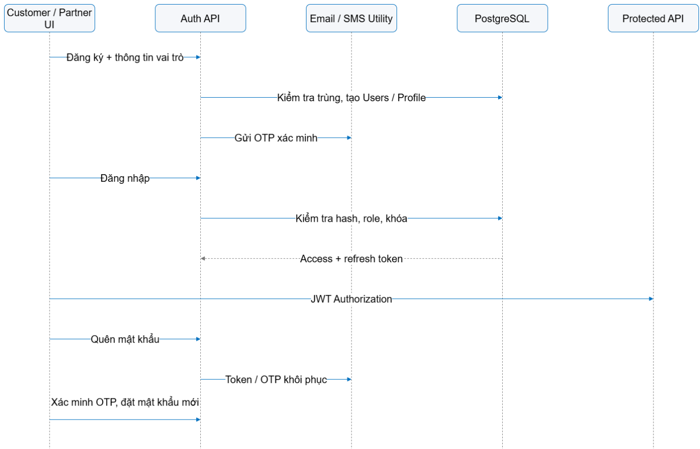
Hình 3.7: Sequence diagram cho đăng ký, đăng nhập, JWT và khôi phục mật khẩu
