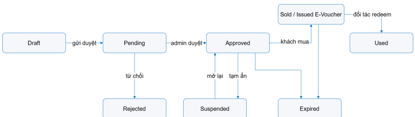
Hình 3.11: State diagram vòng đời voucher và E-Voucher
