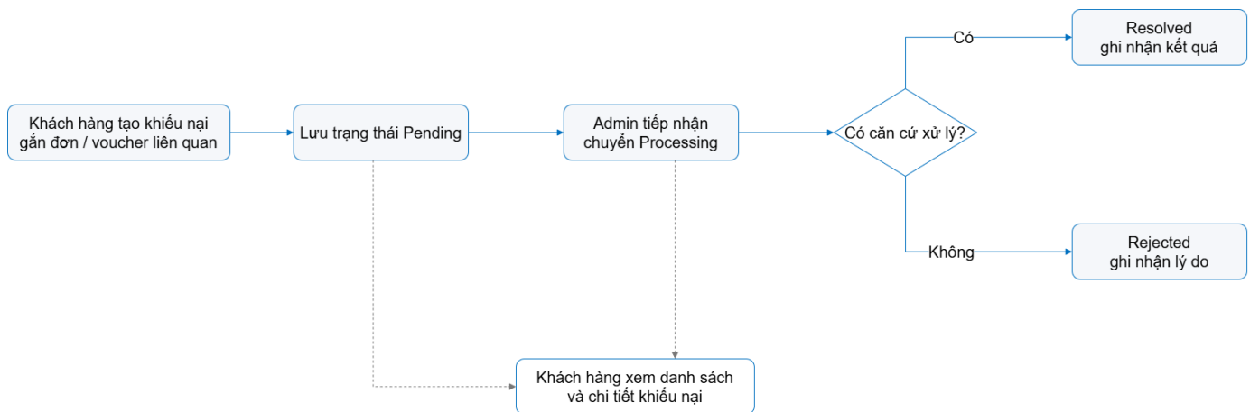
Hình 3.5: Activity diagram cho tiếp nhận, xử lý và theo dõi khiếu nại
