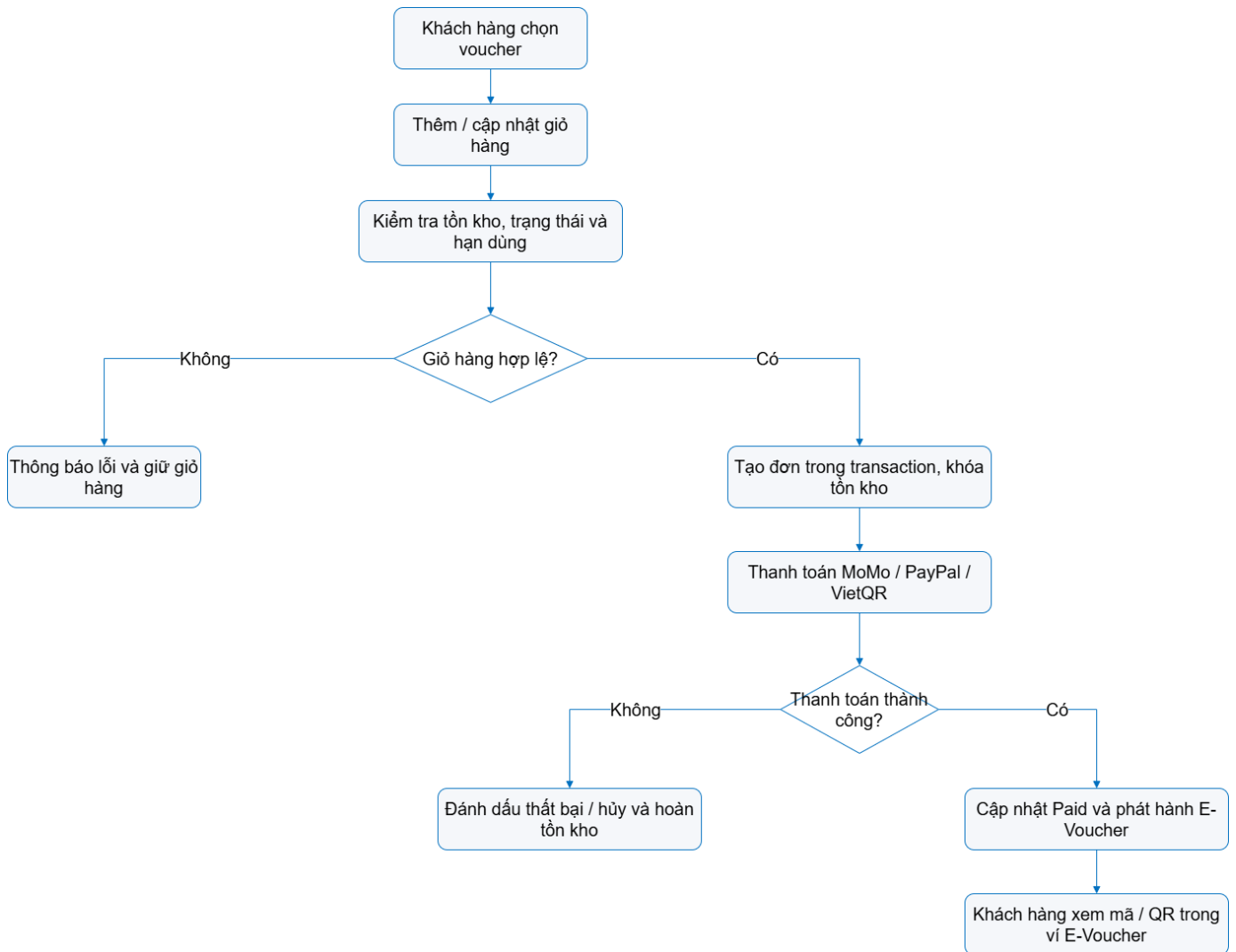
Hình 3.4: Activity diagram cho quá trình mua và phát hành E-Voucher
