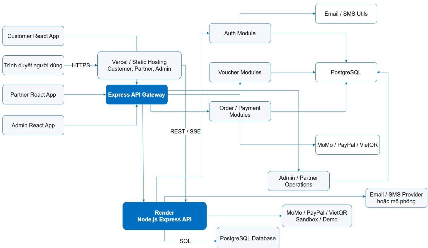
Hình 3.15: Deployment diagram mức triển khai demo
