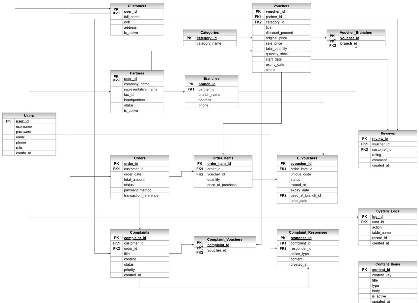
Hình 3.16: ERD hệ thống voucher
