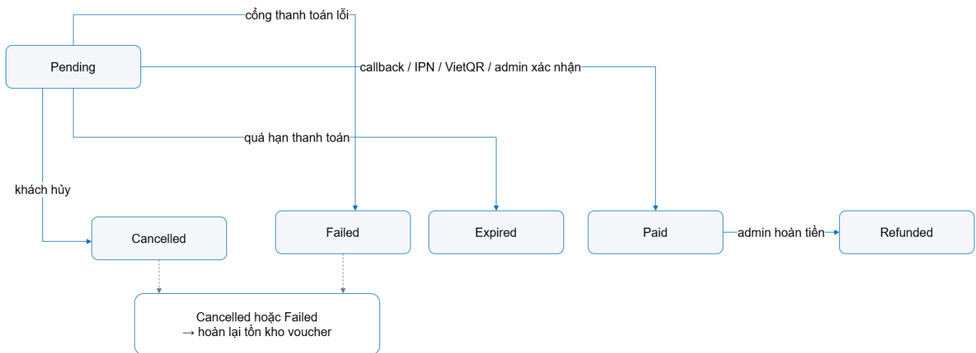
Hình 3.12: State diagram vòng đời đơn hàng và các nhánh hoàn tồn kho
