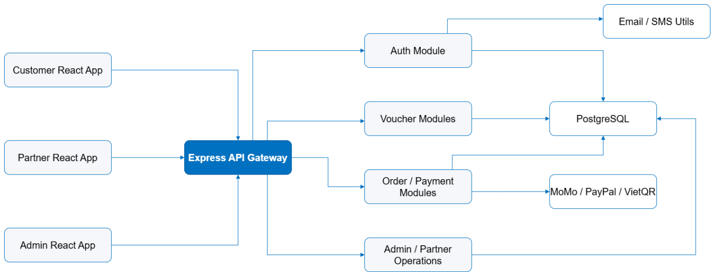
Hình 3.14: Component diagram của hệ thống
