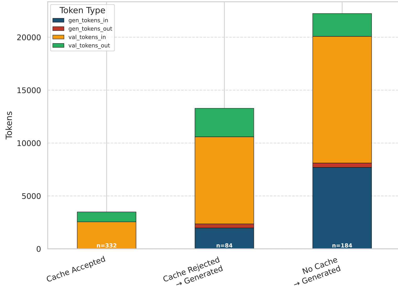
Token Cost per Scenario
