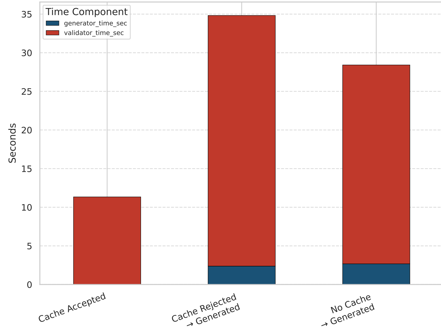
Time Cost per Scenario
