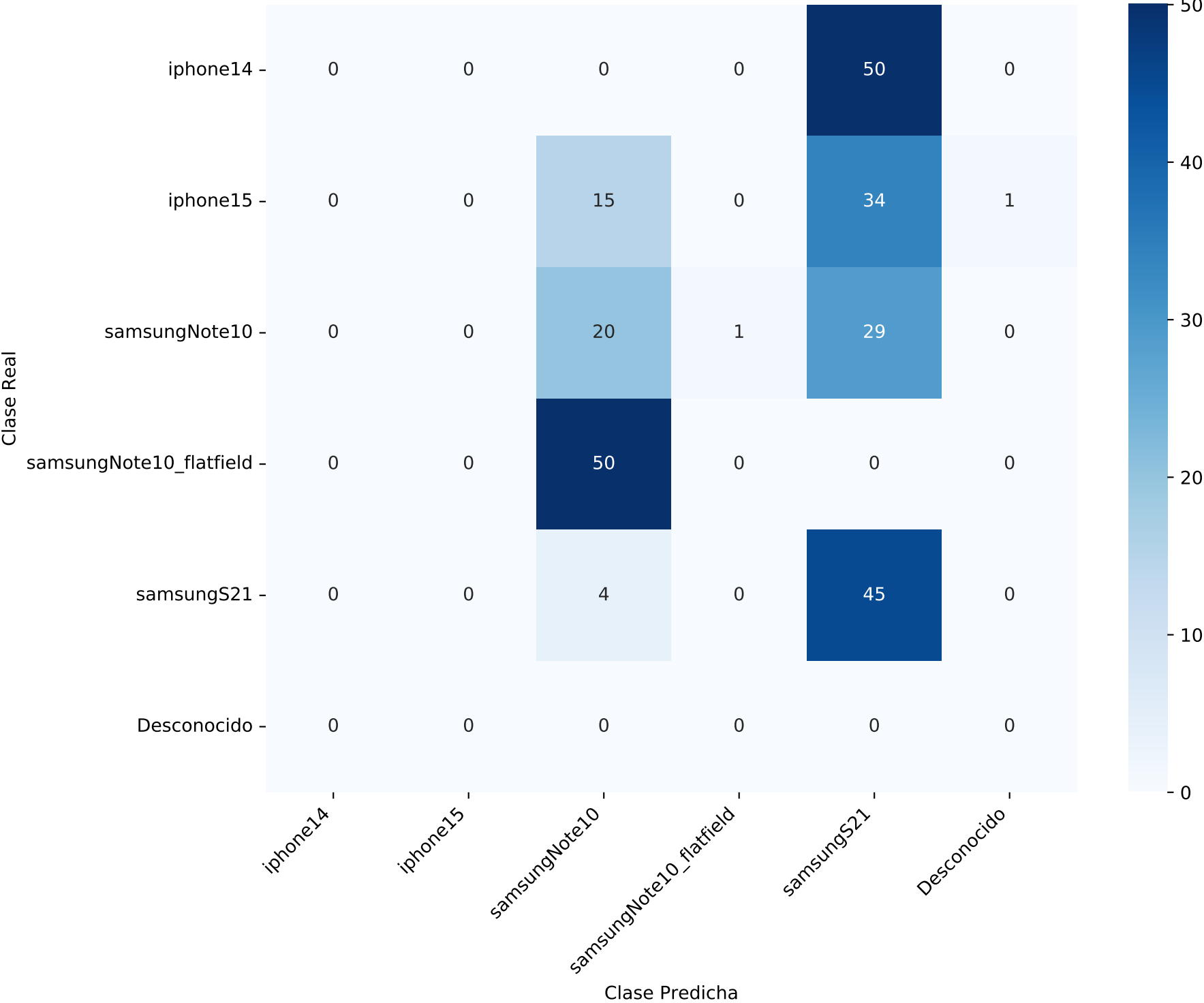
Matriz de Confusión - NOISEPRINT_WHATSAPP
