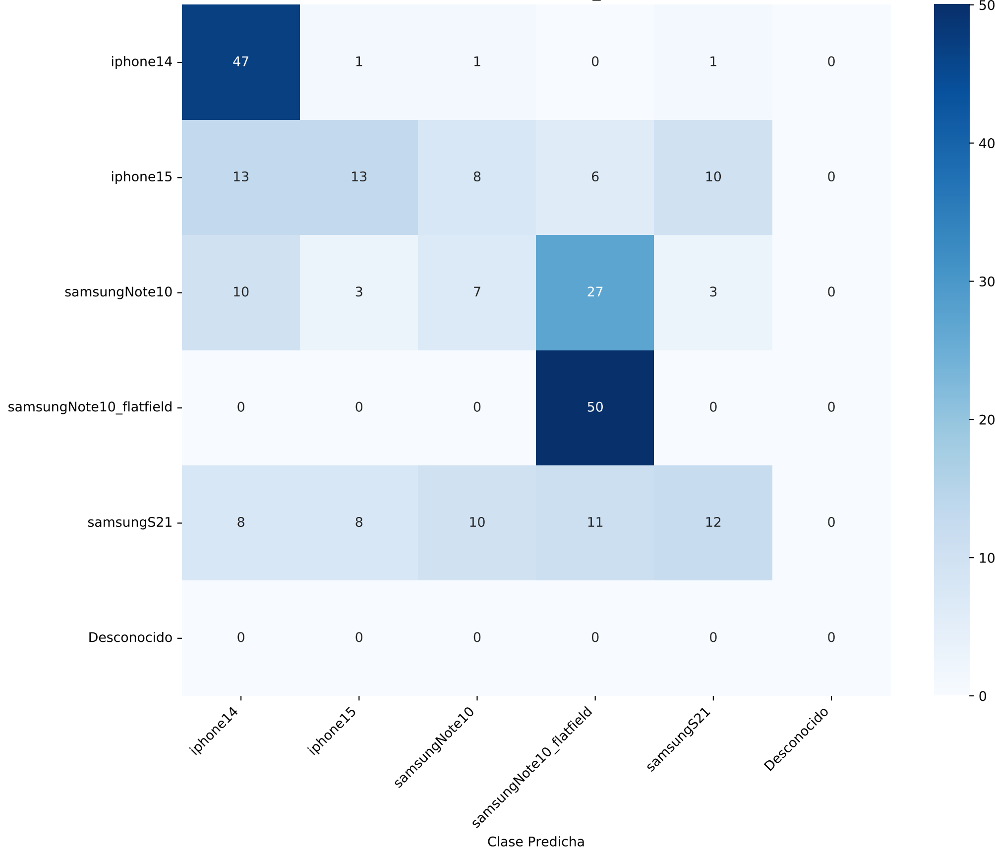
Matriz de Confusión - PRNU_ORIGINALES
