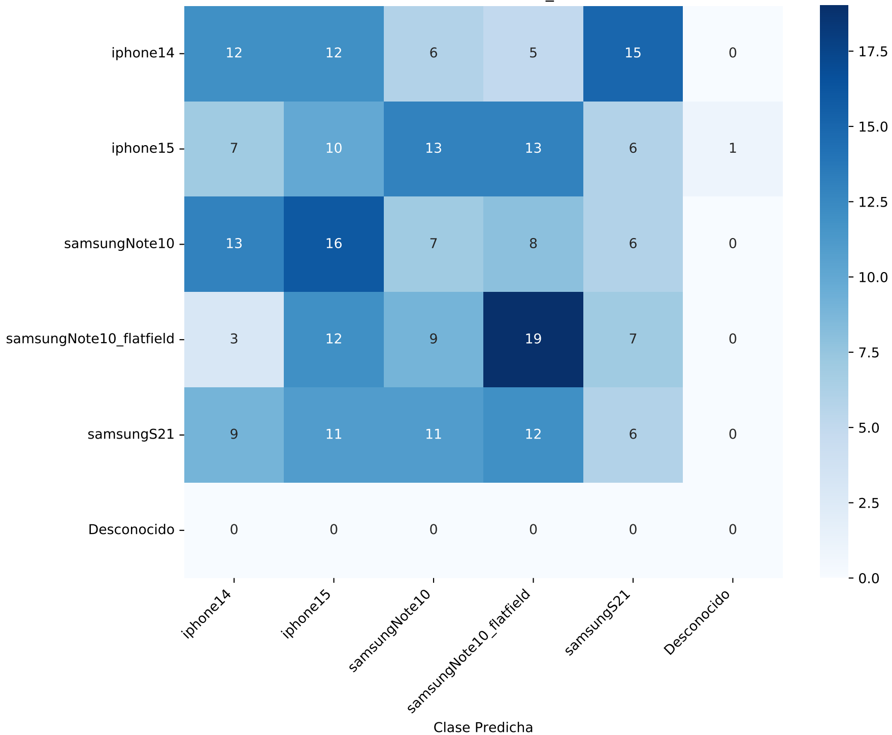
Matriz de Confusión - PRNU_WHATSAPP
