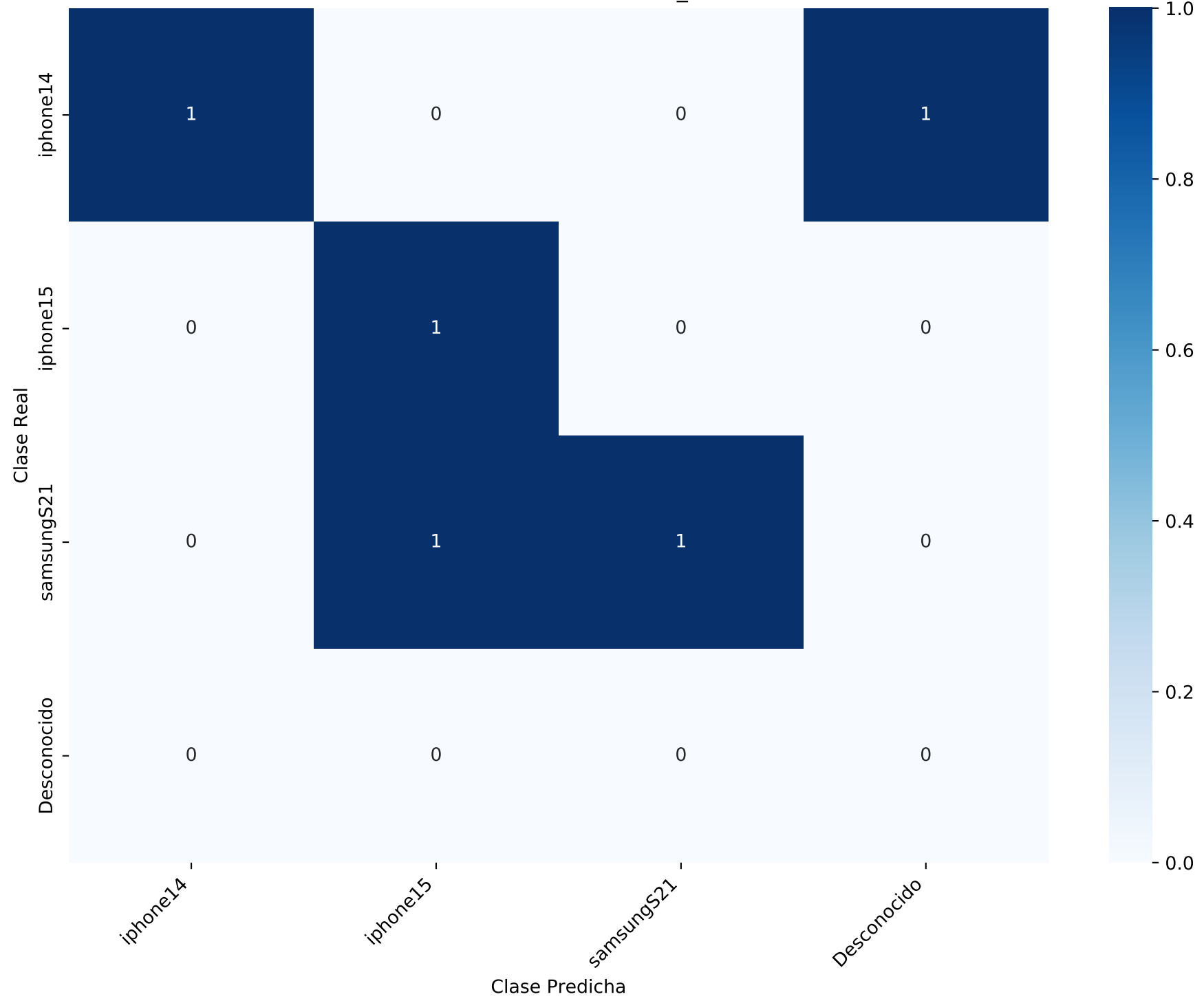
Matriz de Confusión - PRUEBA_RAPIDA
