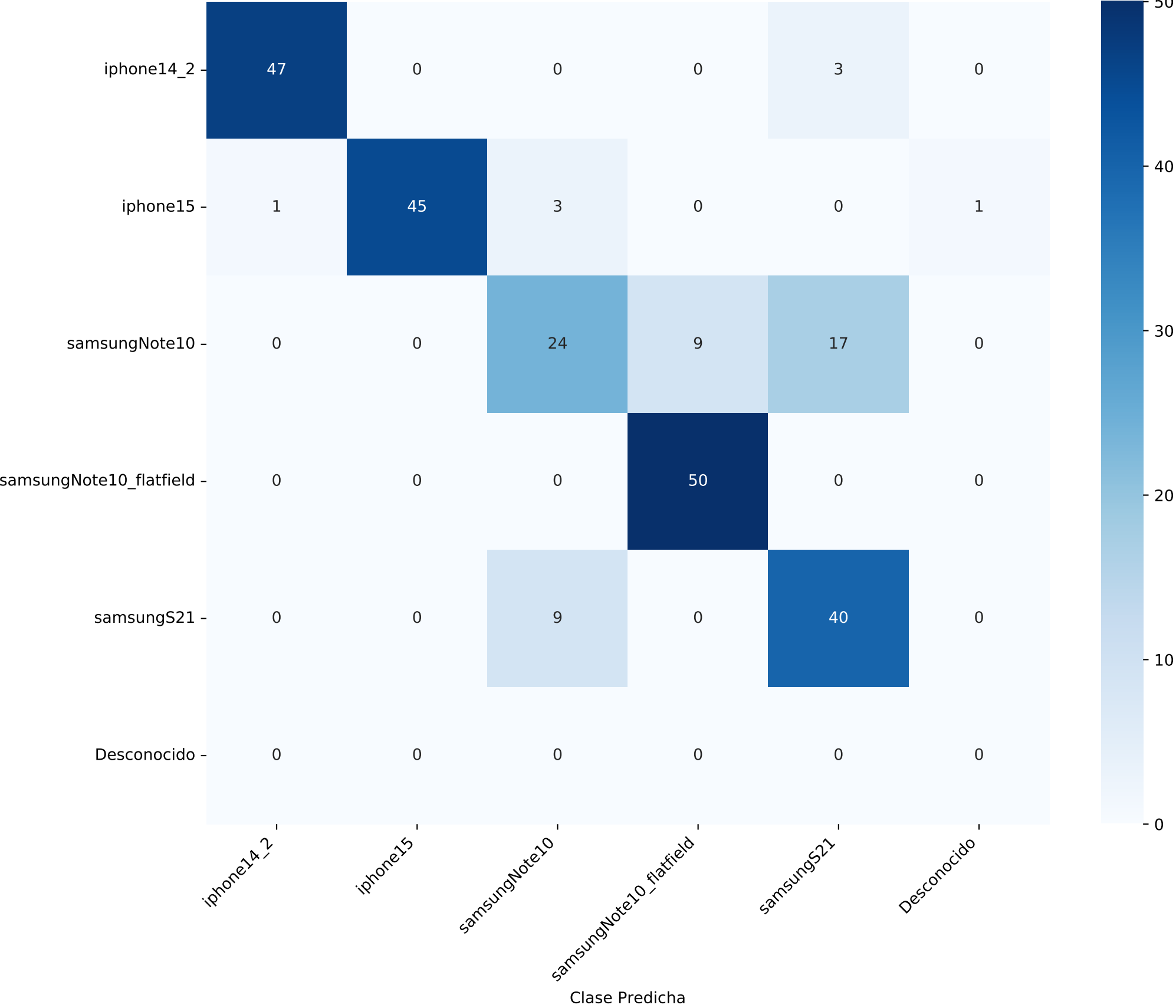
Matriz de Confusión - NOISEPRINT_ORIGINALES
